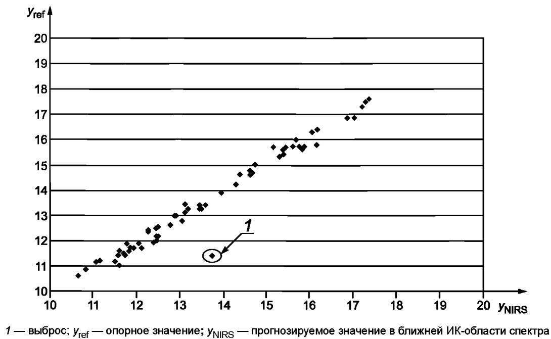
Рисунок В.4 — График рассеяния с y -выбросом
