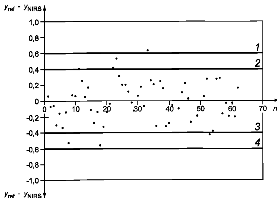
1 — верхняя граница действия (UAL, +3s_{SEP} ); 2 — верхняя предупредительная граница (UWL, +2s_{SEP} ); 3 — нижняя граница предупредительная (LWL, -2s_{SEP} ); 4 — нижняя граница действия (LAL, -3s_{SEP} ); n — номер измерения; y_{ref} — опорное значение; y_{NIRS} — прогнозируемое значение в ближней ИК-области спектра
