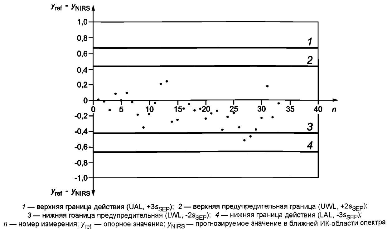
Рисунок В.6 — Контрольная карта для определения содержания жира в зерне, %
