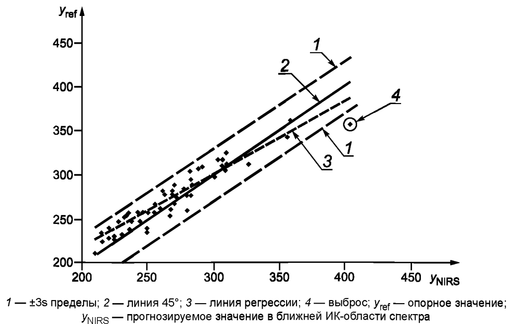
Рисунок В.5 — Пример определения ADF в зерне на кормовые цели с у-выбросом
