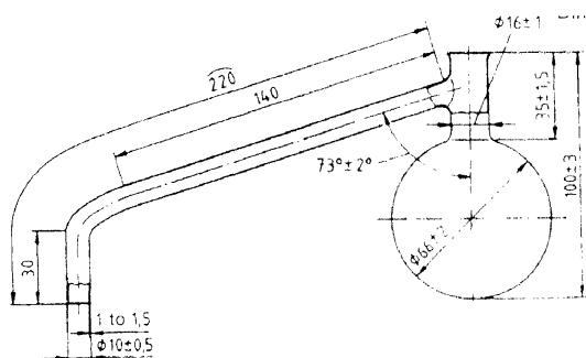
Рисунок 2 – Перегонная колба для определения содержания твердого парафина
