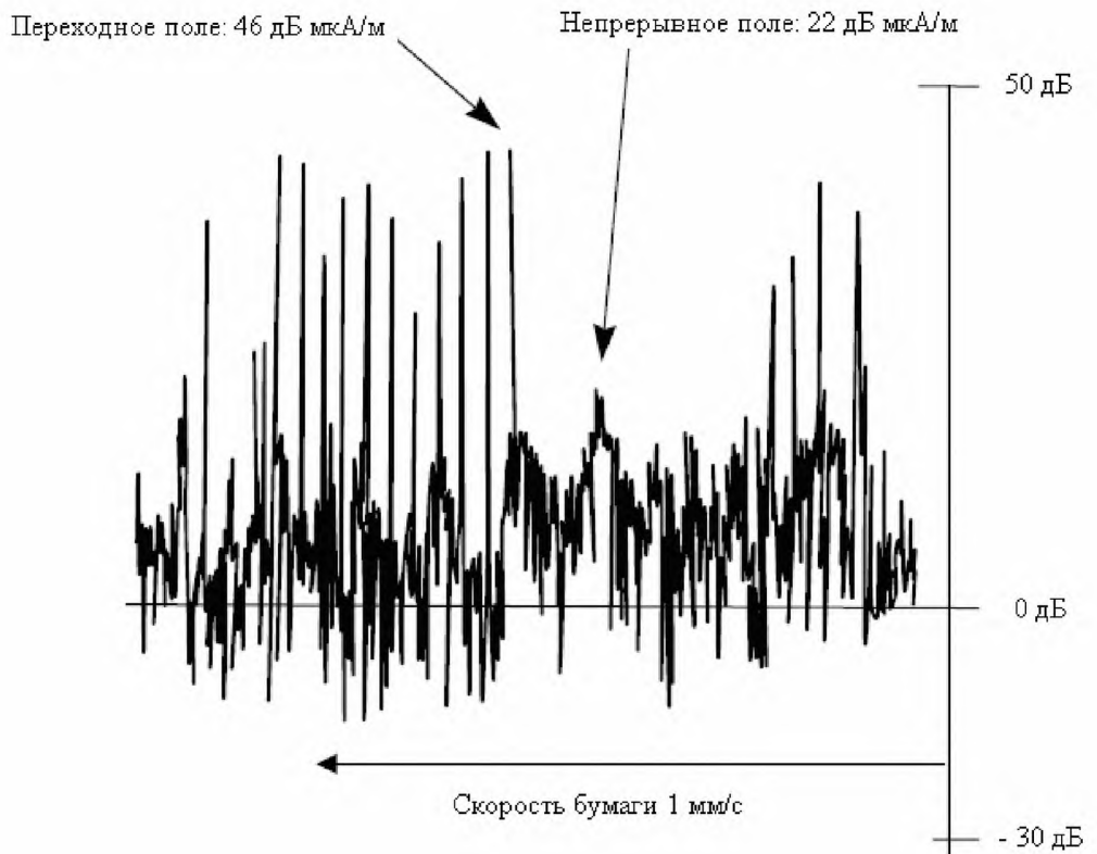
Рисунок Б.1 – Изменение во времени излучений, производимых движущимся поездом с образованием многочисленных переходных полей
