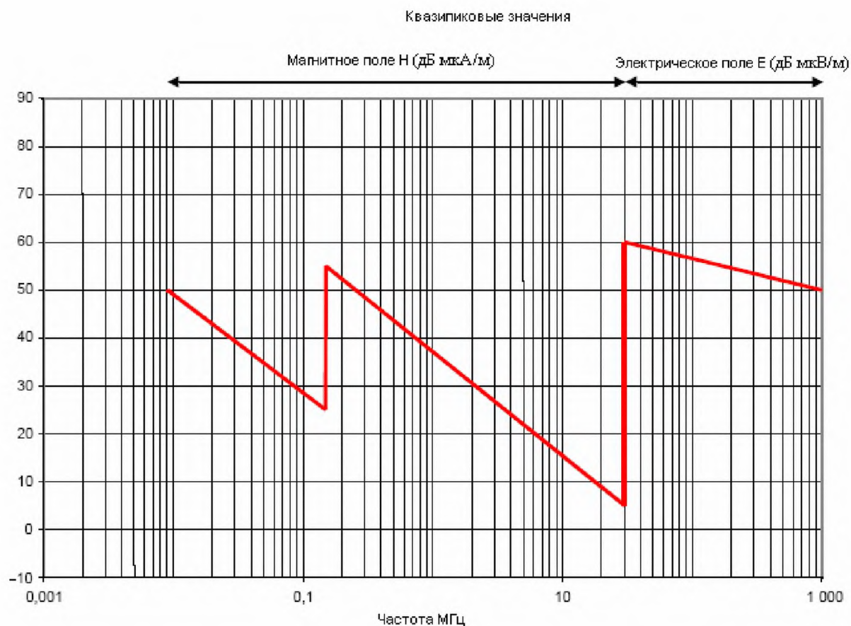
Рисунок 2 – Пределы излучений тяговых подстанций
