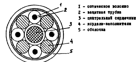
СХЕМЫ КОНСТРУКЦИЙ СЕРДЕЧНИКОВ ОК
