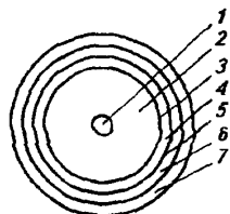
Рис. 1. Радиочастотный коаксиальный кабель
