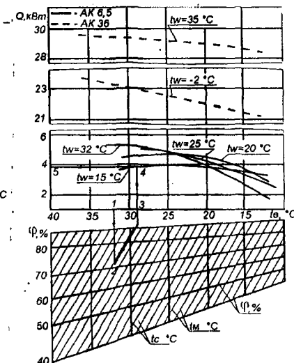
Графики теплотехнических характеристик кондиционеров АК 6,5, АК 36
