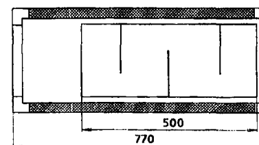
Шумоглушитель m = 21 \text{ кг}
