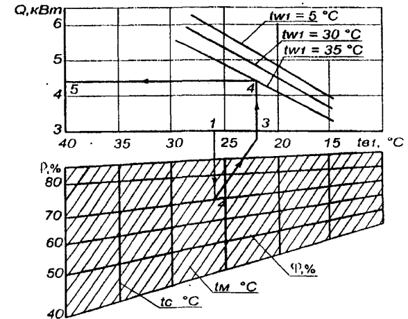
График теплотехнических характеристик кондиционера в режиме охлаждения
