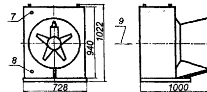
Конденсаторная секция
