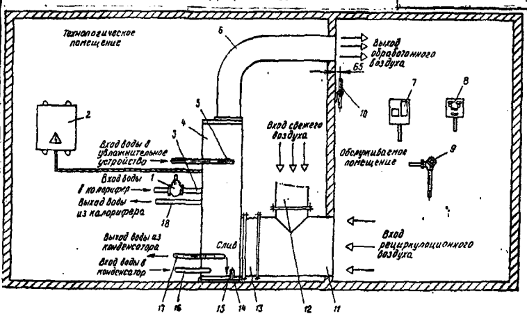
СХЕМА УСТАНОВКИ КОНДИЦИОНЕРА КПА1
