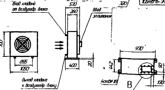
Блок конденсаторный (наружный)
