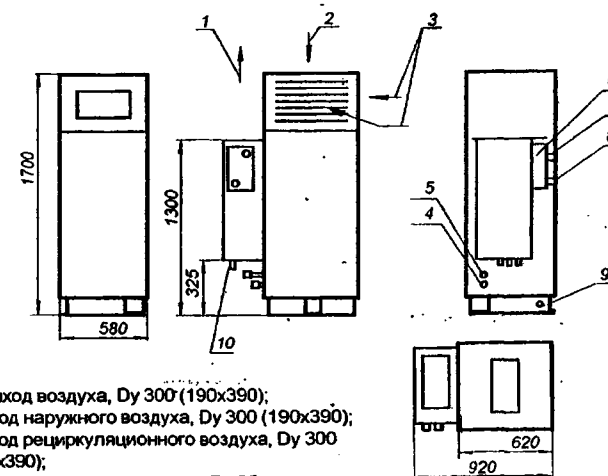
Кондиционер автономный АК 18, АКП 18 (левая модель)
