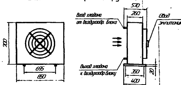
Блок конденсаторный (наружный)
