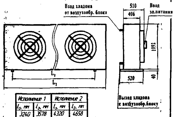
Блок конденсаторный (наружный)
