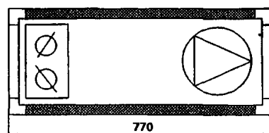
Моноблок 3 Состав: воздухозаборный клапан, вентилятор, фильтр ФЯ m = 36 \text{ кг}
