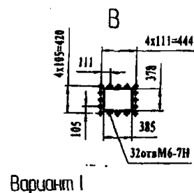
Блок конденсаторный (наружный)
