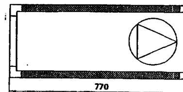
Моноблок 4 Состав: воздухозаборный клапан, вентилятор, фильтр ФЯ, воздухонагреватель водяной, m = 43 \text{ кг}
