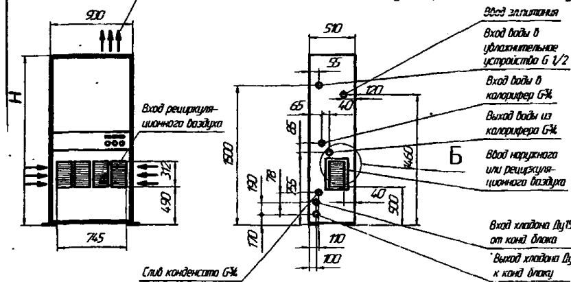
Блок воздухообрабатывающий (внутренний)
