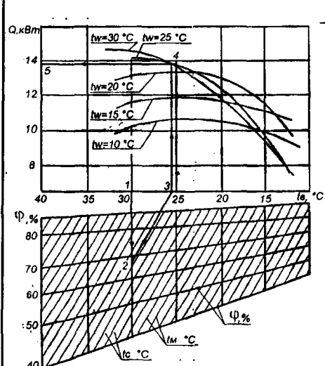
Графики теплотехнических характеристик кондиционеров АК 18/6, АК 18, АКЛ 18
