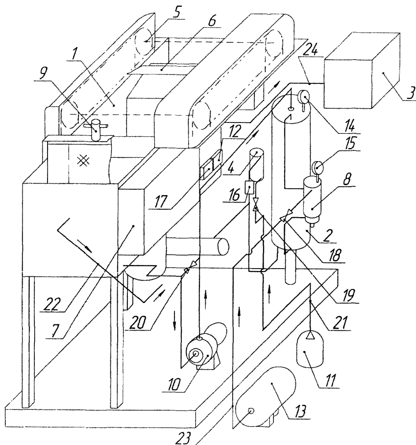
Схема установки "ФМН 2 O+" принципиальная
