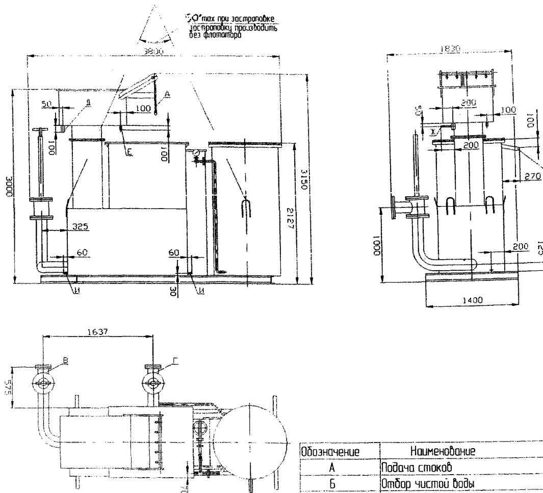
Общий вид установки "Береза"
