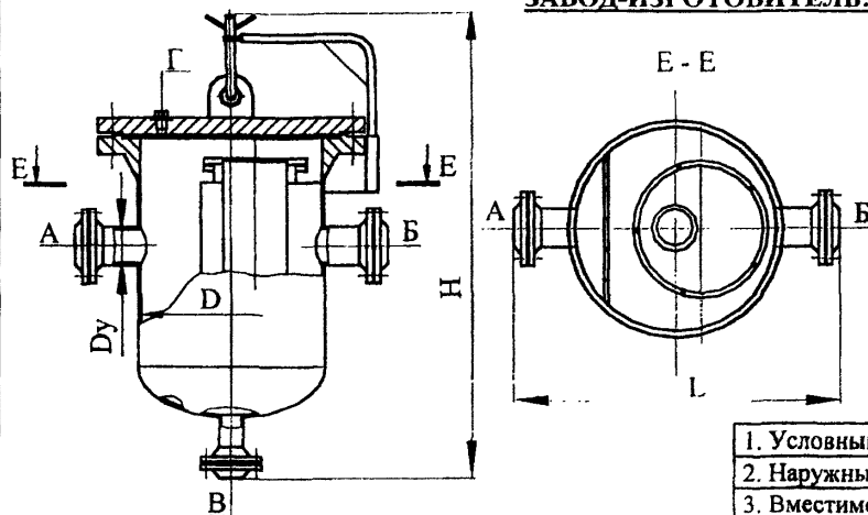
Характеристика штуцеров
