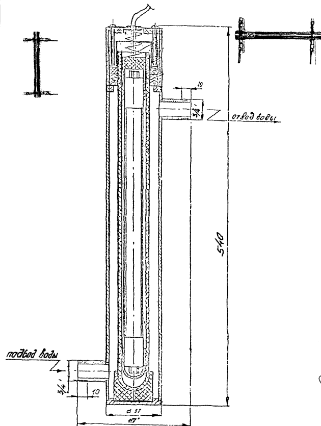
БАКТ-1
