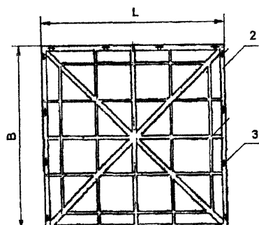
БЛОК ВОДОУЛОВИТЕЛЯ
