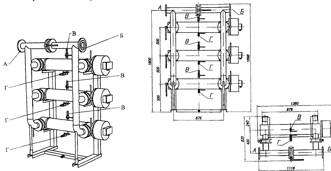
Блок бактерицидного обеззараживания ББО-60
