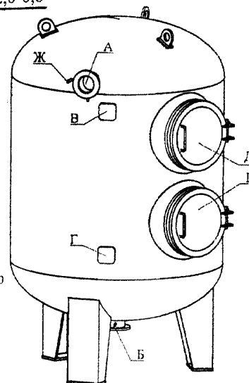
ФОВ-2,0-0,6
