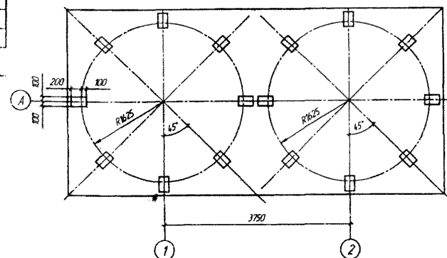
Монолитная плита основания ПМ1
