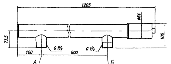
БАКТ-5
