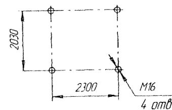
План расположения фундаментных болтов
