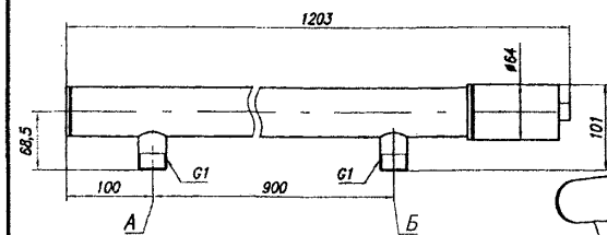
БАКТ-3
