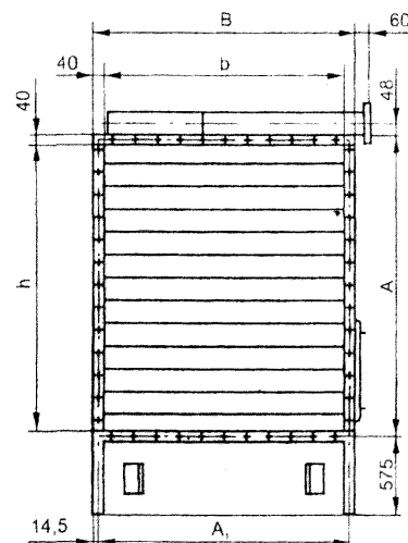
А - для ГФВС-31,5; ГФВС-40
