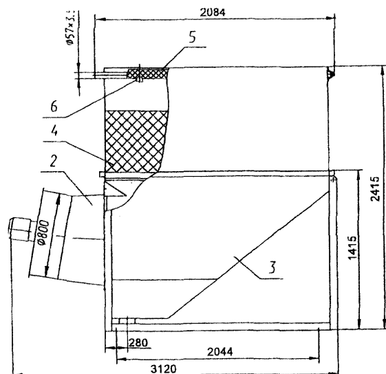
ГРД-24, ГРД-32
