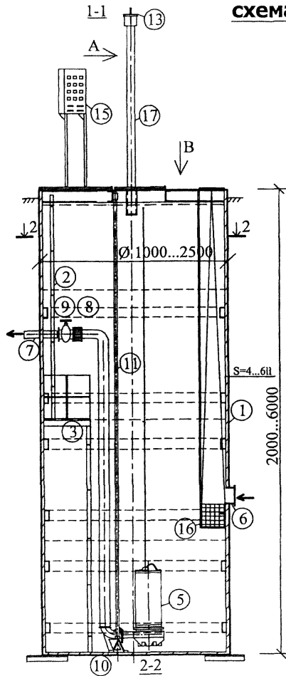
схема КНС
