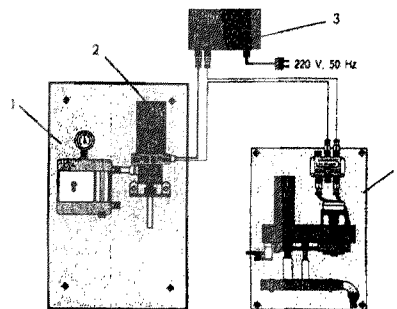
1 - хлоратор АХВ-1000/Е; 2 - ЭМДВ; 3 - блок питания; 4 - АСХВ.
