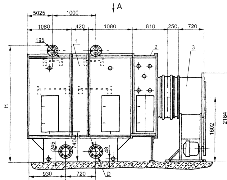
А - для ГФВС-60; ГФВС-80
