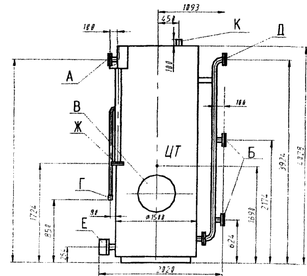
Фильтр ИНСТЭБ-2,8
