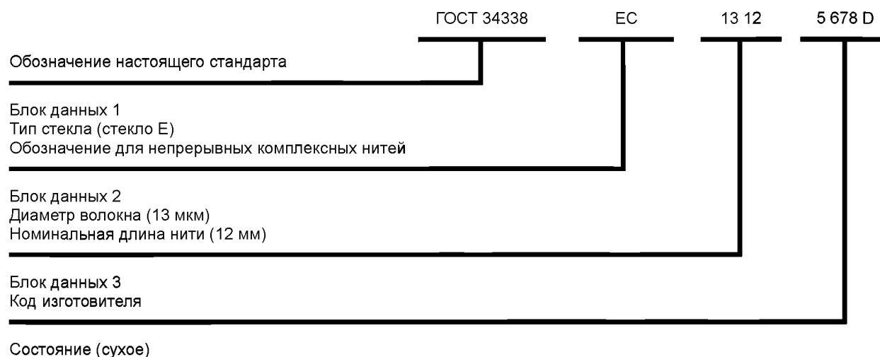
Рисунок 3 — Обозначение ГОСТ 34338-ЕС, 13 12, 5 678 D
