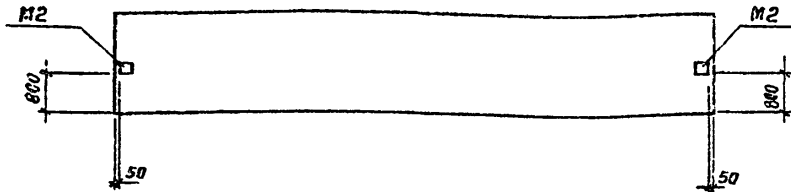
Изделие закладное М2 установить по данному чертежу
