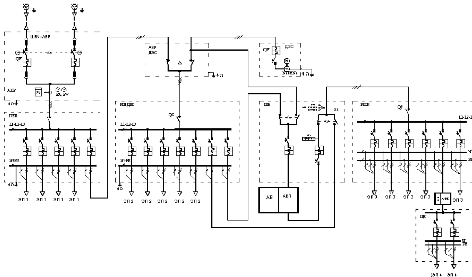
Рисунок J.8 – Пример принципиальной электрической схемы комбинированного питания здания (сооружения) с преимущественным применением ЭККП
