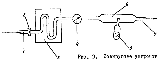
Рис. 3. Дозирующее устройство
