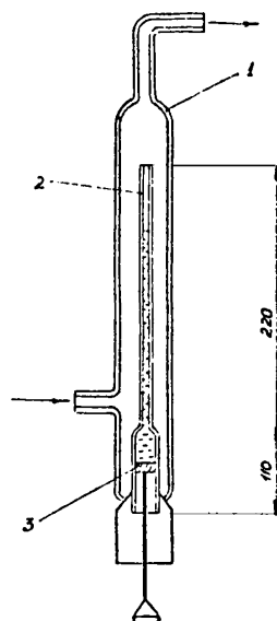
Рис. 1. Дозирующее устройство
