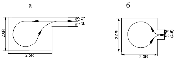
Рисунок 6 – Разворотные площадки на тупиковых внутриобъектных дорогах:
