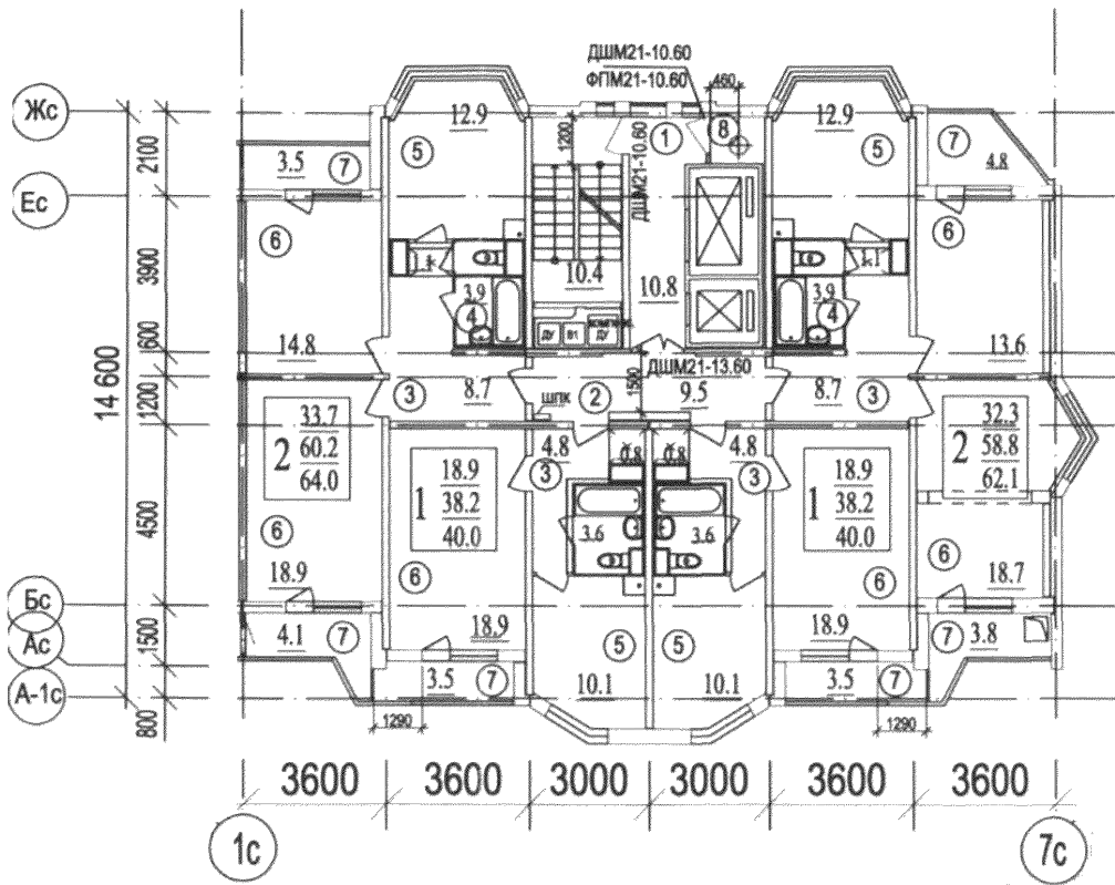
Рисунок Б.2 – Типовой этаж торцевой блок-секции типового жилого дома П44
