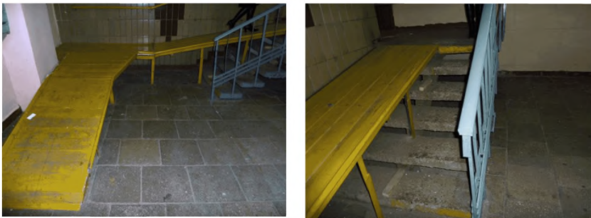
Рисунок 6.2.14 – Пандус в габаритах вестибюля жилого дома
