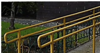
Рисунок 6.1.21 – Недопустимые конструкции креплений поручней на пандусе
