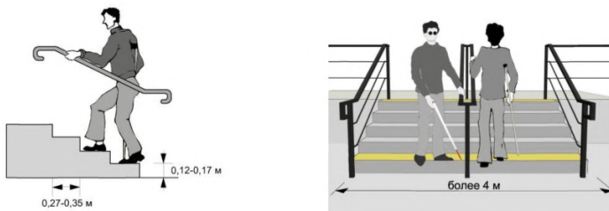
Рис.6.1.10, а – Ступени единой геометрии и поручни на широких лестницах
