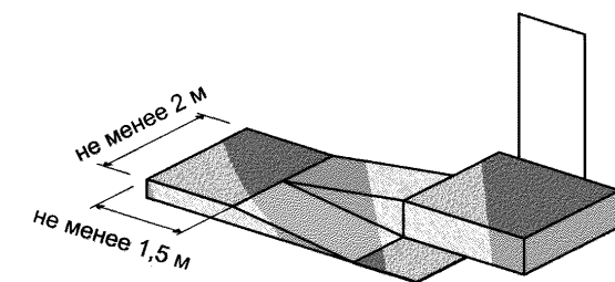
П-образный пандус
