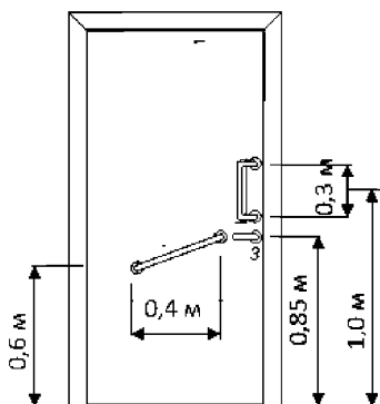
Рисунок 6.5.16 – Расположение ручки и задвижки на двери
