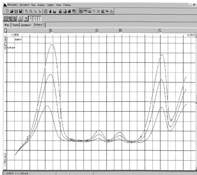
Рисунок 8. Вольтамперограммы фоновое электролита, пробы и пробы с добавками АС элементов при одновременном определении цинка, кадмия, свинца и меди
