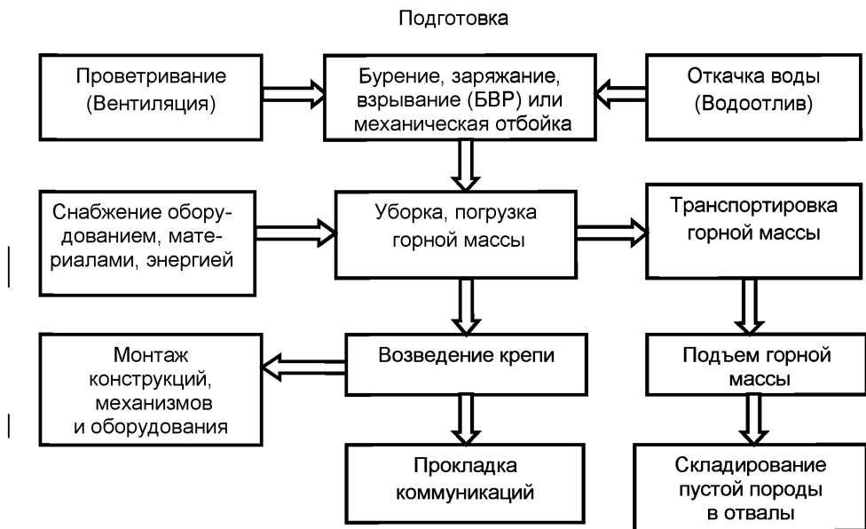
Рисунок 2.3 — Общая блок-схема процессов подготовительных работ
