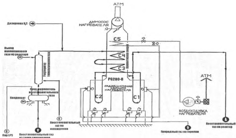
Рисунок 2.47 — Нагреватель восстановительного газа
