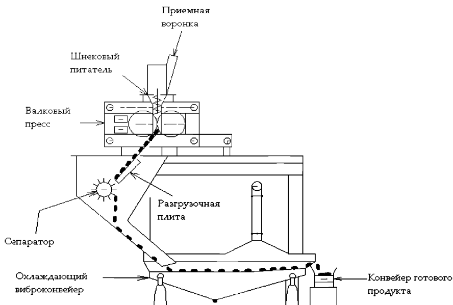
Рисунок 2.50 — Схема установки брикетирования и охлаждения брикетов
