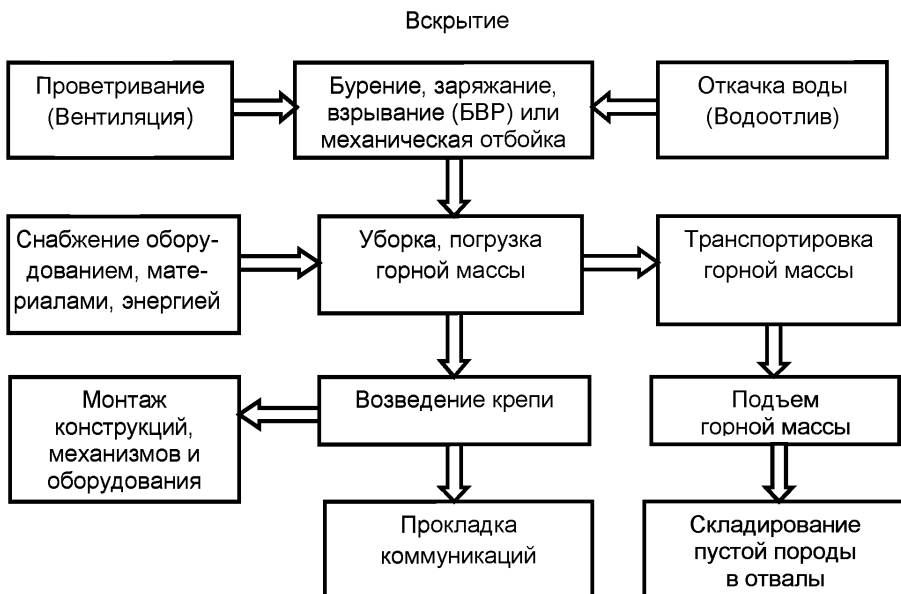
Рисунок 2.2 — Общая блок-схема процессов этапа вскрытия
