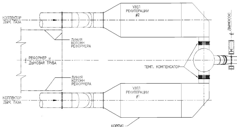
Рисунок 2.48 — Схема системы рекуперации тепла на установках MIDREX
