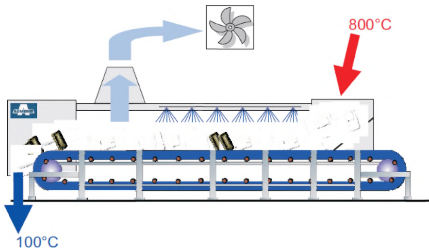
Рисунок 2.51 — Принцип действия конвейера медленного охлаждения
