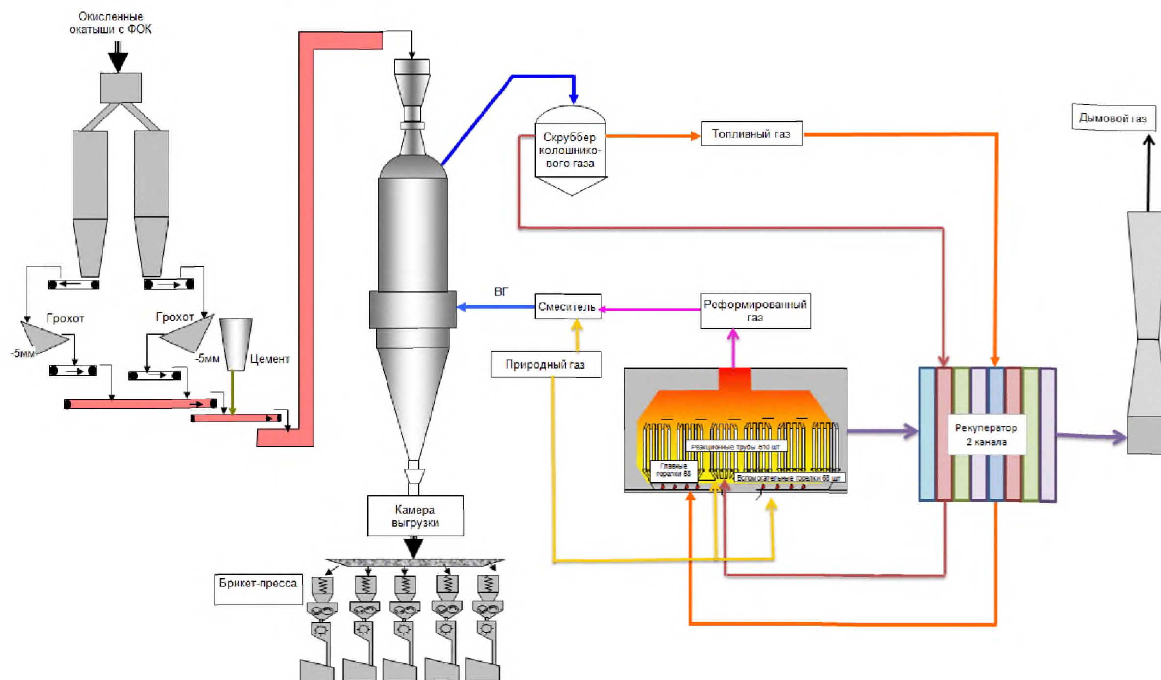
Рисунок 2.34 — Технологическая схема MIDREX
