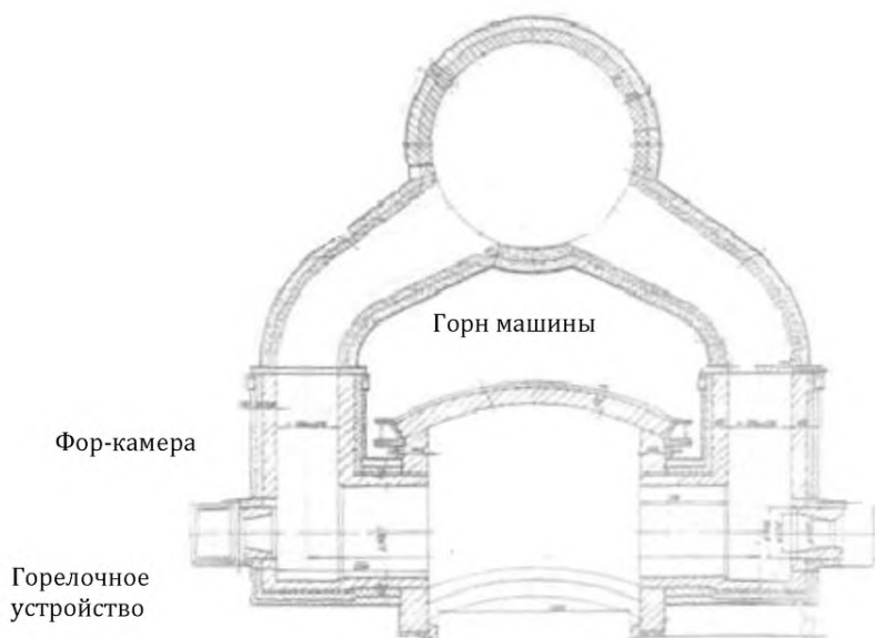
Рисунок 2.27 — Поперечное сечение горна обжиговой машины
