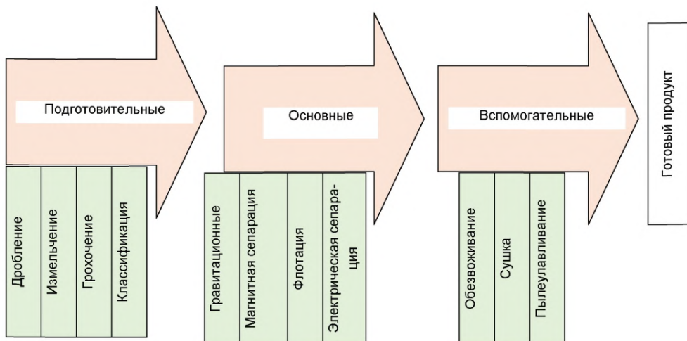
Рисунок 2.6 — Обобщающая схема технологического процесса обогащения
