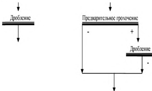
Рисунок 2.8 — Схемы одностадийного дробления в открытом цикле
