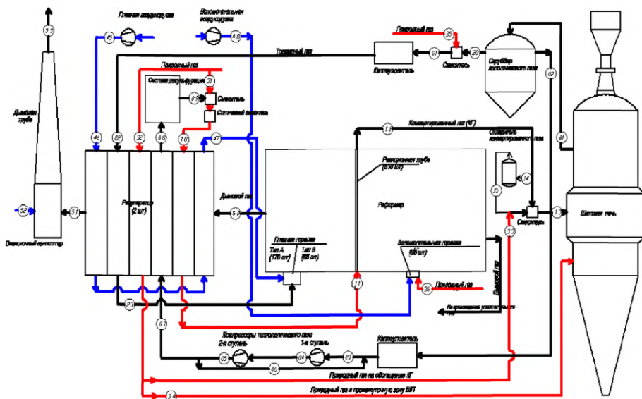
Рисунок 2.45 — Схема потоков технологических газов на установке MIDREX
