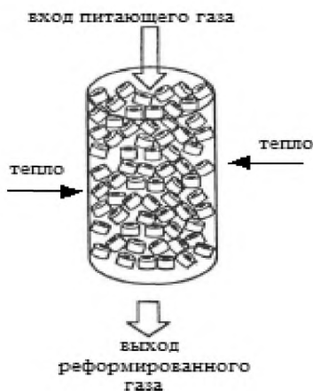
Рисунок 2.42 — Реакционная труба реформера, заполненная катализатором
