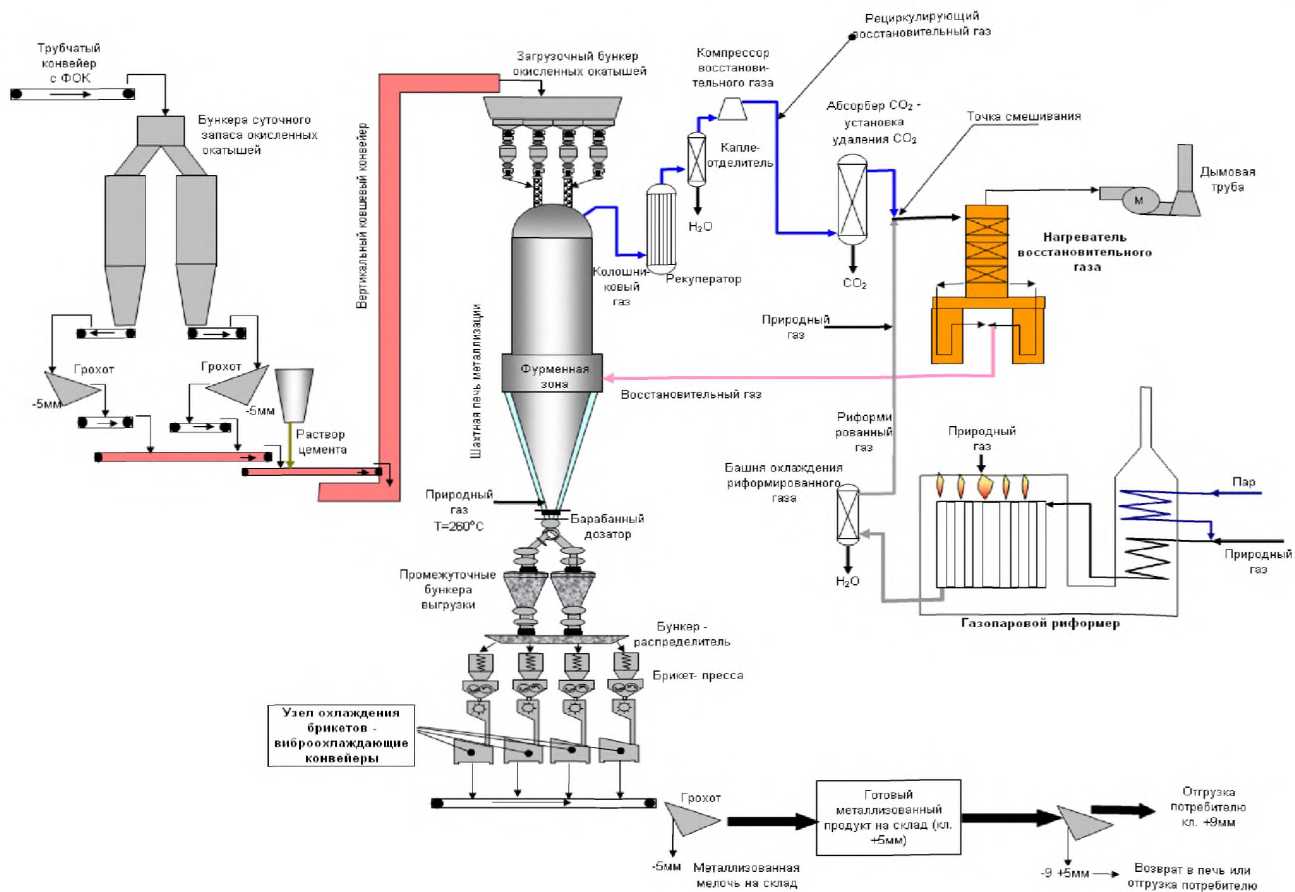
Рисунок 2.33 — Технологическая схема HYL-III
