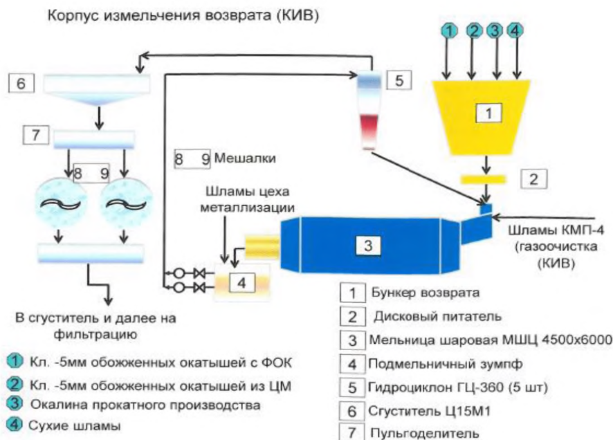
Рисунок 3.6 — Схема использования шламов на ОЭМК.
