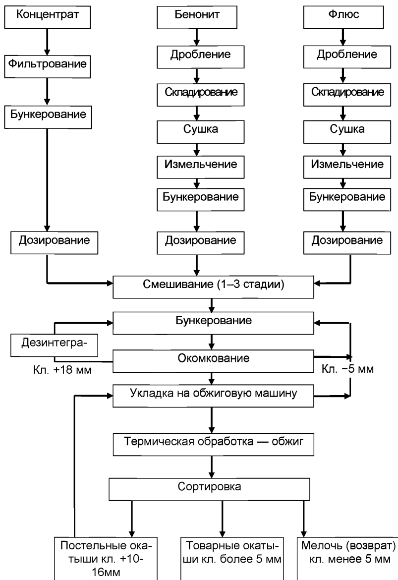
Рисунок 2.15 — Обобщенная структурная схема производства окатышей
