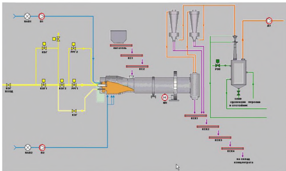
Рисунок 2.13 — Типовая схема сушки концентрата
