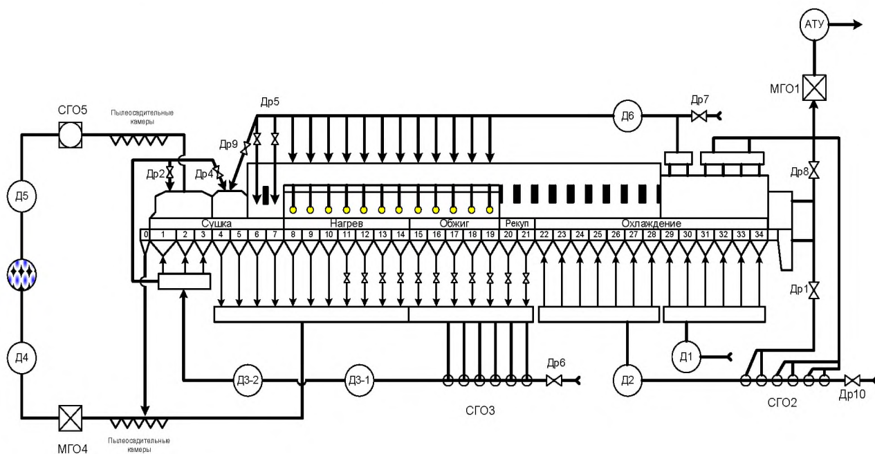
Рисунок 2.21 — Тепловая схема действующей модернизированной ОК-228
