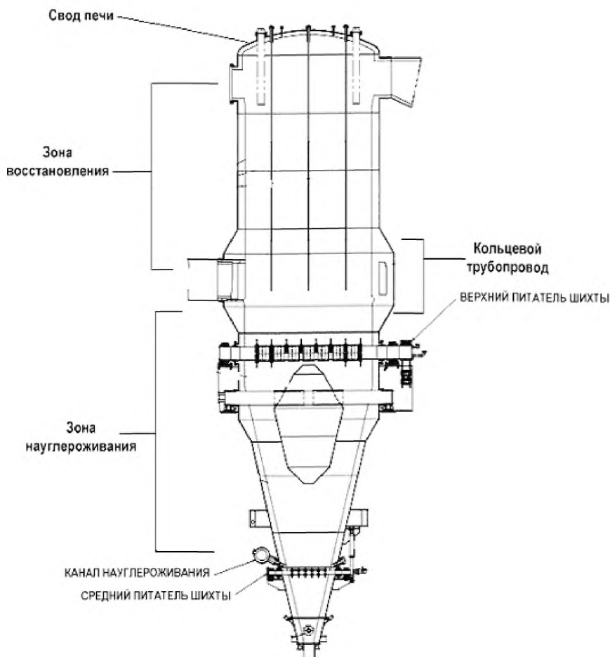
Рисунок 2.37 — Общий вид шахтной печи металлизации MIDREX
