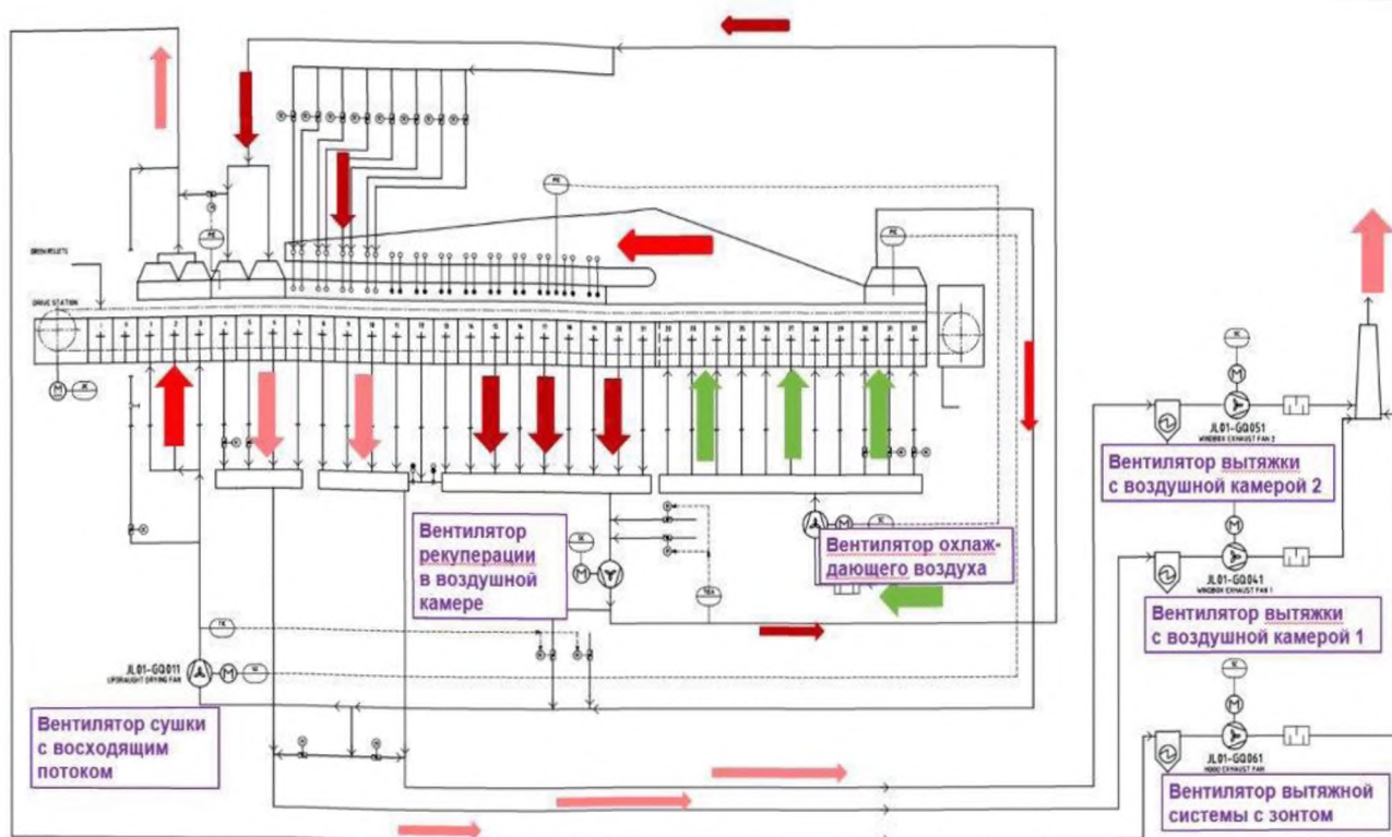
Рисунок 2.26 — Схема газовых потоков обжиговой машины О-768
