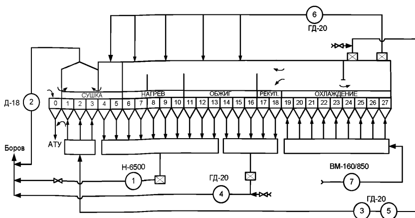
Рисунок 2.20 — Тепловая схема действующей ОК-108
