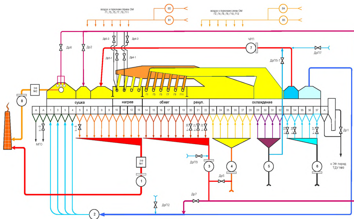
Рисунок 2.24 — Схема газовых потоков обжиговой машины МОК-1-592М
