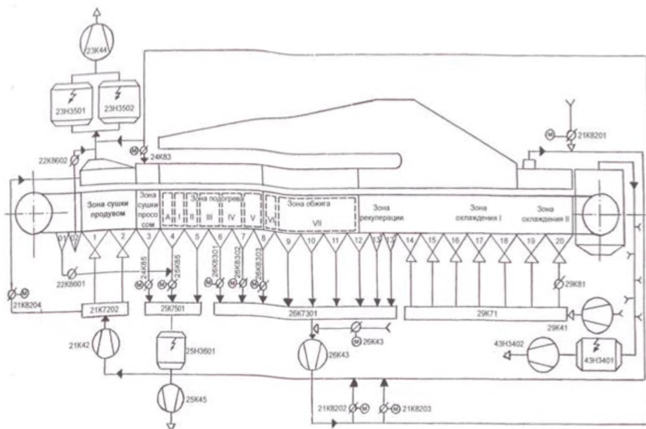
Рисунок 2.25 — Схема газовых потоков обжиговой машины Л-480
