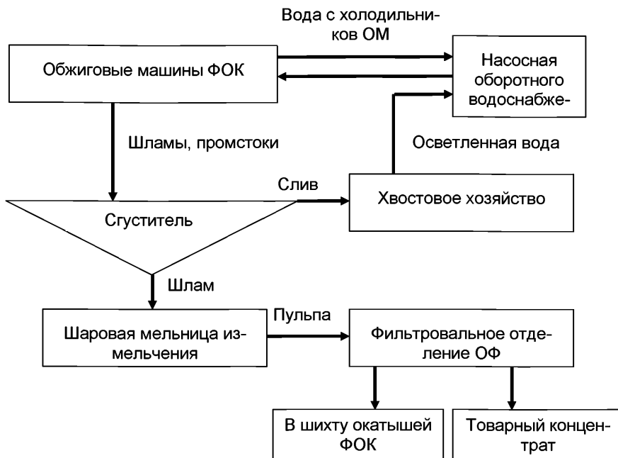
Рисунок 2.31 — Обобщенная схема движения шламов фабрик окомкования
