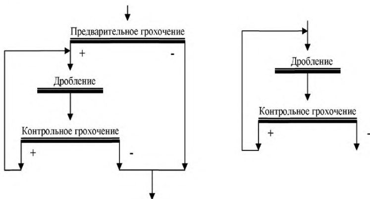
Рисунок 2.9 — Схемы одностадийного дробления в замкнутом цикле
