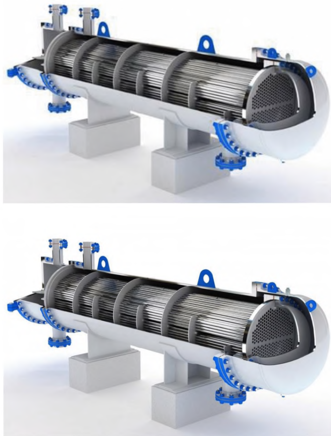
Рисунок 2.46 — Кожухотрубный противоточный рекуператор технологического газа
