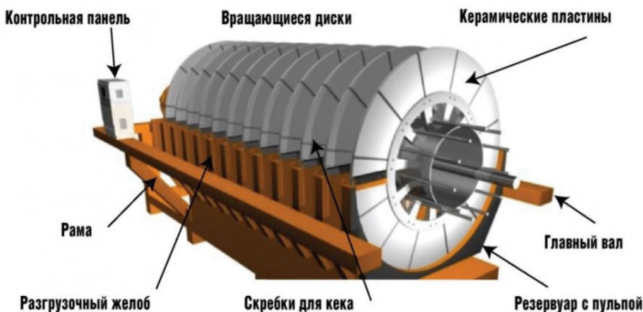
Рисунок 2.12 — Дисковый вакуумный фильтр
