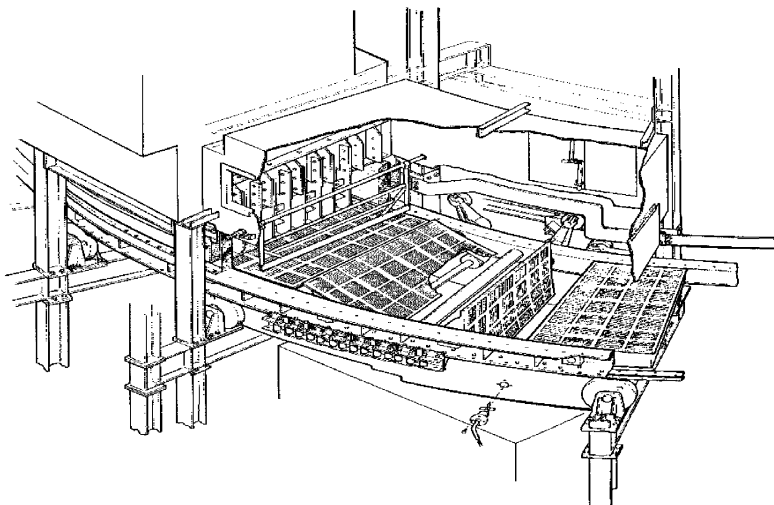
Рисунок 2.30 — Кольцевой охладитель
