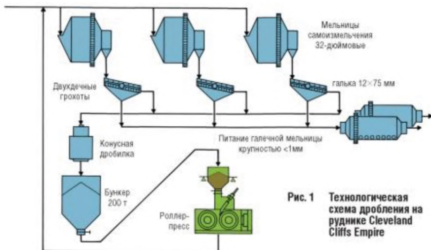
Рисунок 7.9 — Пример размещения роллер-пресса в технологии самоизмельчения
