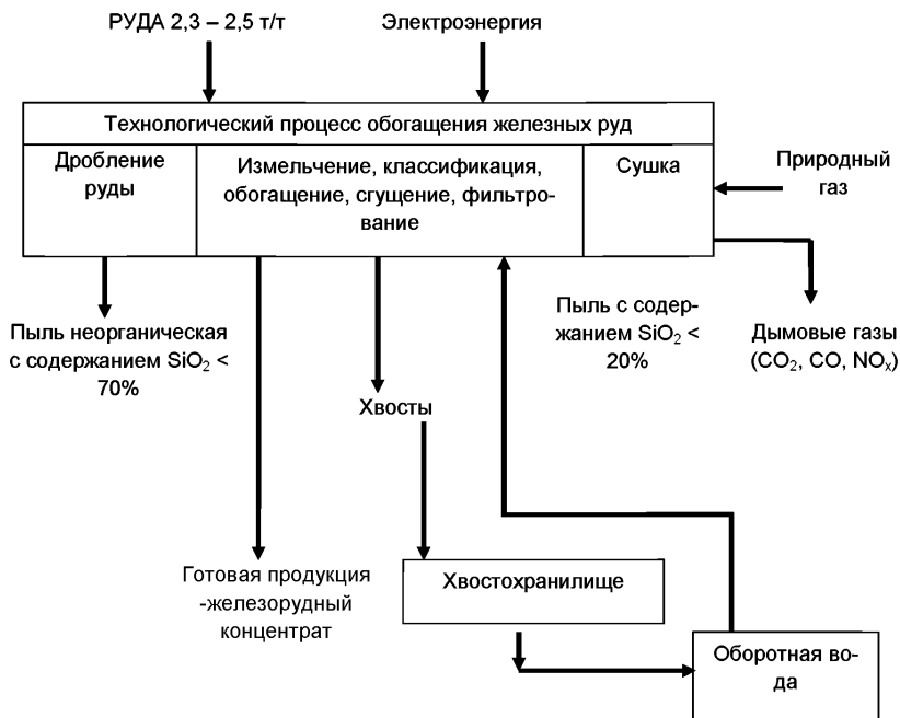
Рисунок 3.5 — Обобщенная схема движения шламов фабрик окомкования.
