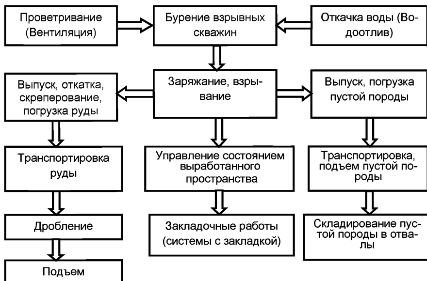
Рисунок 2.4 — Общая блок-схема процессов очистных работ
