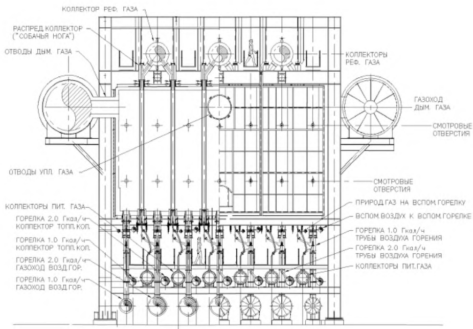
Рисунок 2.41 — Реформер установки MIDREX. Вид с торца
