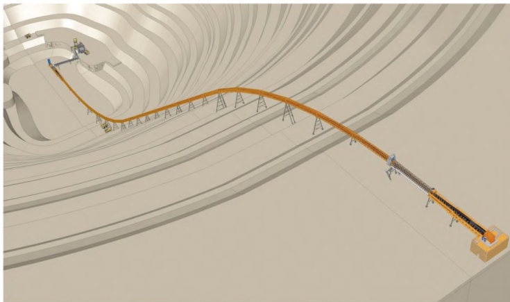
Рисунок 7.2 — Трехмерная схема крутонаклонного конвейера из карьера
