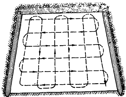
Рис. 8. Схема обвода поперечного сечения выработки анемометром
