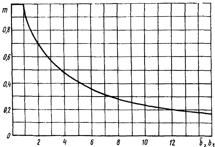
Рис. 8. Величина коэффициента m для точечных источников, размещенных на крыше отдельно стоящего здания в наветренной циркуляционной зоне \left(\bar{b} = \frac{b}{H_{\text{зд}}}\right) и вне этой зоны \left(\bar{b}_3 = \frac{b_3}{H_{\text{зд}}}\right)
