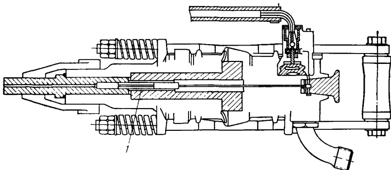
Рис. 50. Закрытие водяной трубки пластиковым шпелем 1
