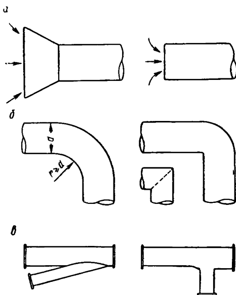
Рис. 100. Примеры правильного (слева) и неправильного (справа) конструктивного выполнения труб:
