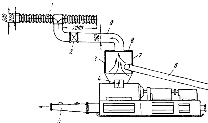
Рис. 41. Пылеулавливание в закладочной машине с ячестым ротором (размеры в миллиметрах):
