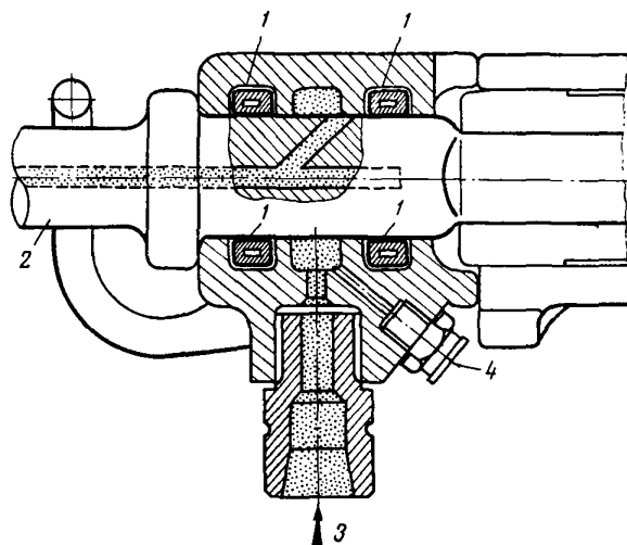
Рис. 51. Устройство для боковой подачи воды:
