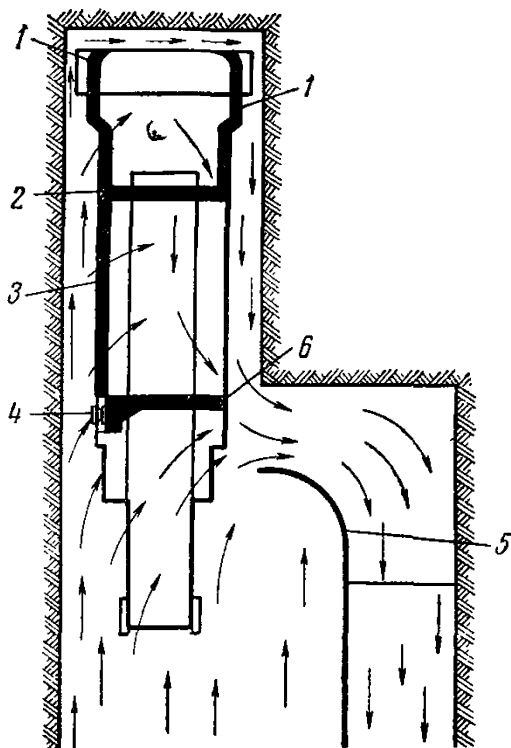
Рис. 26. Вентиляционные трубы, смонтированные на горном комбайне:
