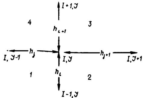
Рис. 1. Схема расположения сеточных узлов для расчета температуры ( t_{i,j} ) и влагосодержания ( u_{i,j} ) для плоского варианта задачи
