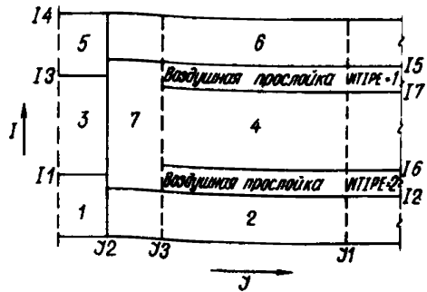
Рис. 2. Схематическое представление исследуемой области для трехслойной панели в области вертикального стыка
