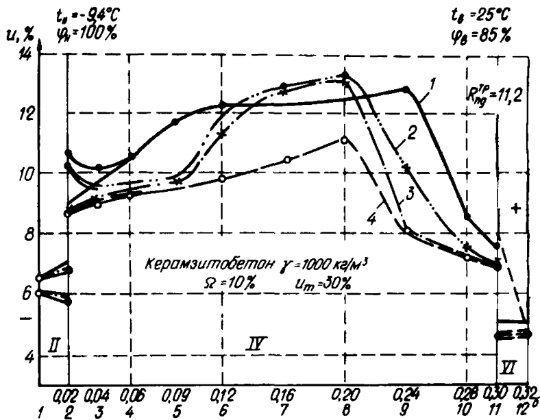
Рис. 17. Влажностное состояние керамзитобетонной панели ( \delta = 0,32 м) с защитным парозащитным слоем ( R_{\text{в}^{\text{п}}} = 11,2 ) в январе, Москва II, VI — цементно-песчаный раствор; IV — керамзитобетон: 1 — первый год эксплуатации; 2 — то же, второй; 3 — то же, третий; 4 — то же, пятый
