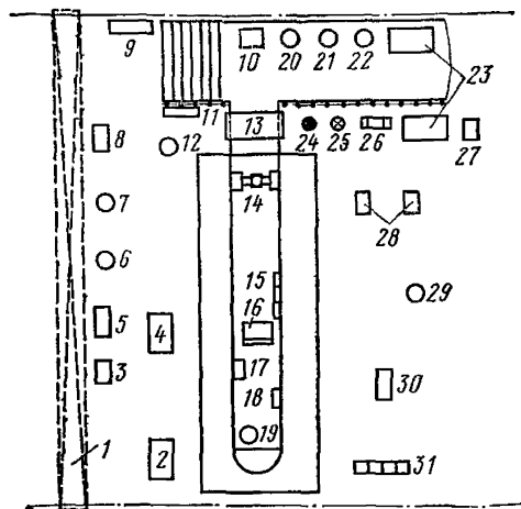
Рис. 1. Схема технологической планировки универсального поста при текущем ремонте автомобилей:
