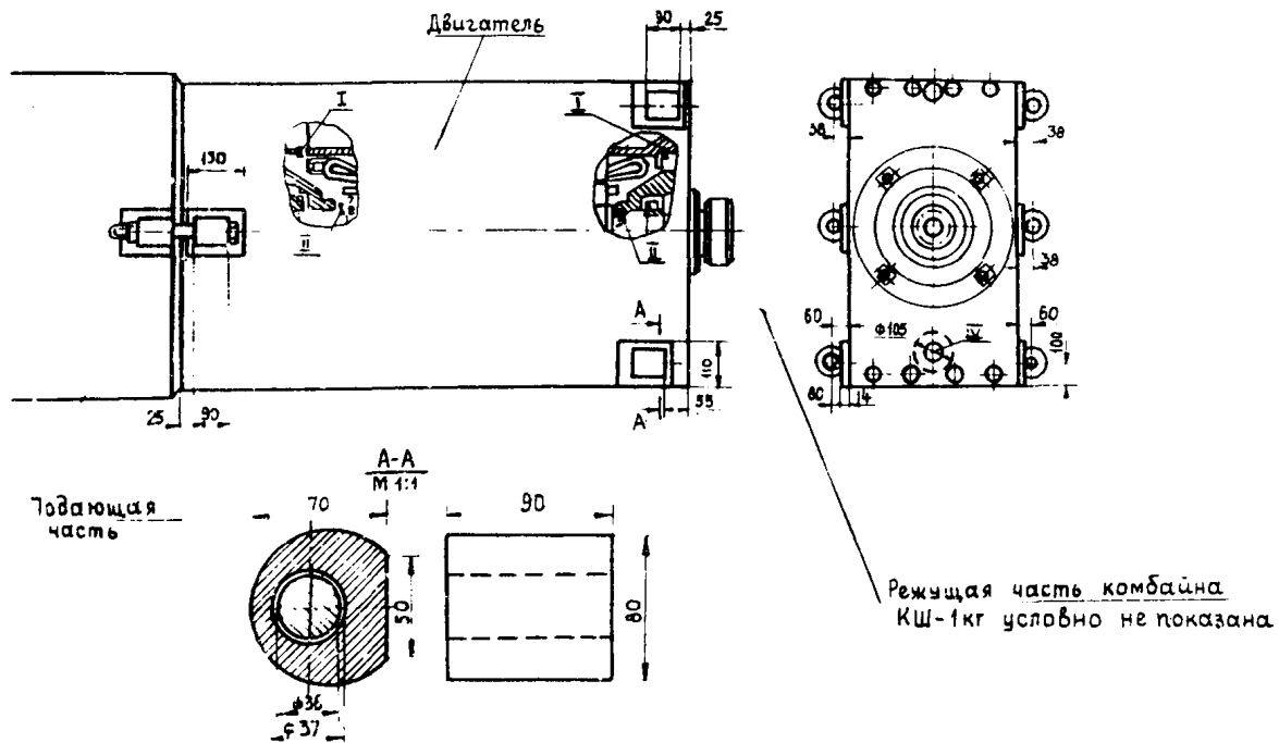
Рис. 2.10. Усиление соединения электродвигателя с подающей и режущей частями комбайна КШ-1кг с помощью дополнительного болтового соединения
