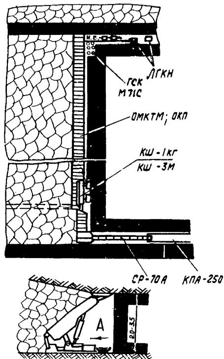
Рис. 3.2. Технологическая схема очистных работ
