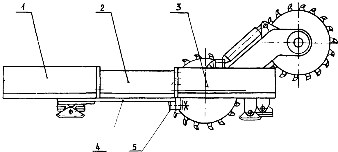
Рис. 2.11. Усиление соединения электродвигателя с подающей и режущей частями комбайна КШ-1КГ с помощью дополнительной стальной плиты: 1 - подающая часть комбайна КШ-1КГ; 2 - электродвигатель; 3 - режущая часть; 4 - плита; 5 - болт М36
