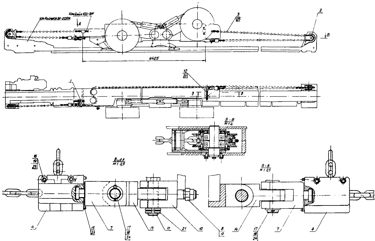
Рис. 2.13. Полиспастная схема механизма подачи Г-405 комбайна КШ-3М
