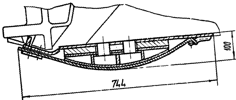
Рис. 2.4. Регулируемая опора секции крени
