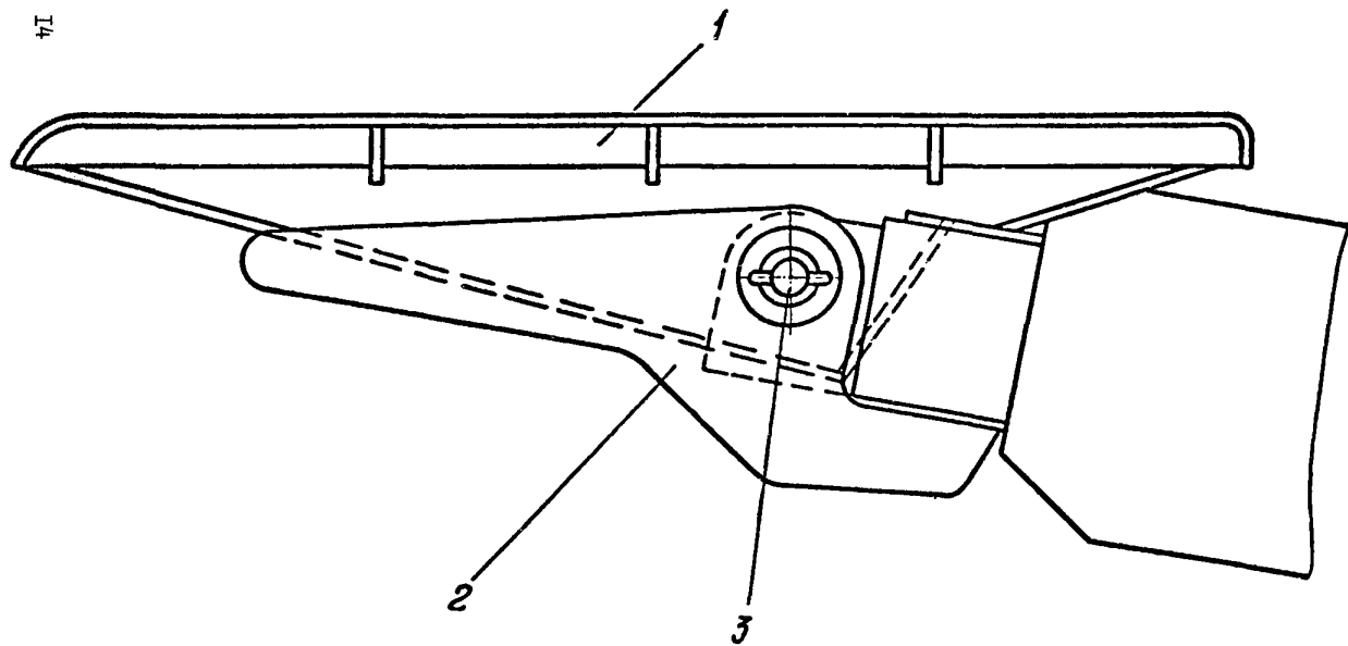
Рис. 2.7. Упорная предохранительная косынка для удержания козырька секции крепи
