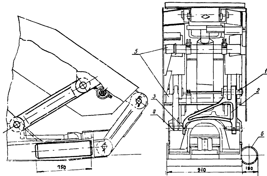
Рис. 2.9. Ограничитель хода выдвижных кожухов секции крени: 1 - ось ОМКТМС-2-003; 2 - рычаг-укосина ОМКТМ-С2-042А; 3 - болт М16; 4 - валик ОМКТМ-С2-002; 5 - ограничитель ОМКТМ-С2-001; 6 - ограни- читель ОМКТМ-С2-000
