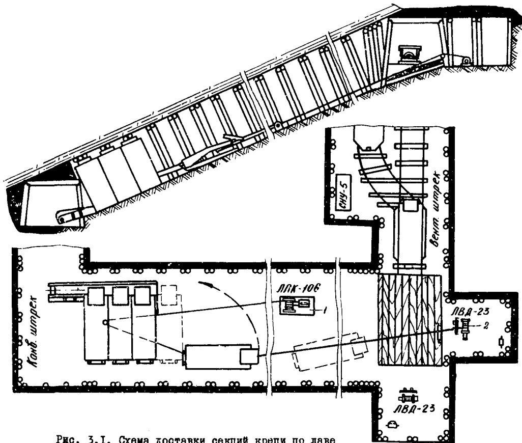
Рис. 3.1. Схема доставки секций крепи по лаве
