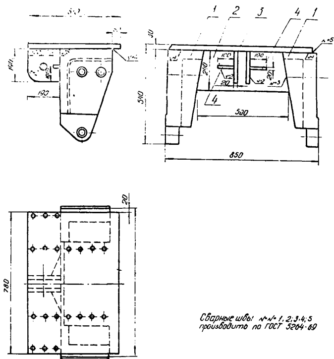
Рис. 2.12. Усиление опор комбайна КШ-1КТ
