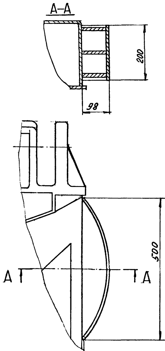
Рис. 2.5. Нерегулируемая опора секции крепи
