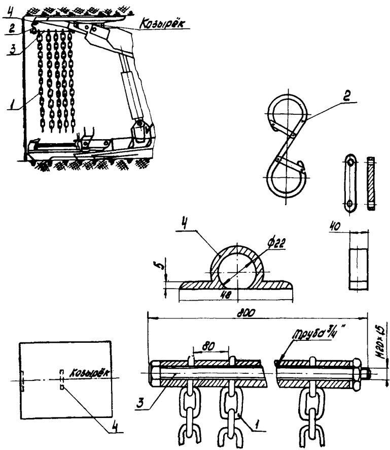
Рис. 1.1. Предохранительный фартук: 1 - цепи; 2 - крючок для подвески цепей; 3 - болт для удержания цепей; 4 - проушина для удержания крючка
