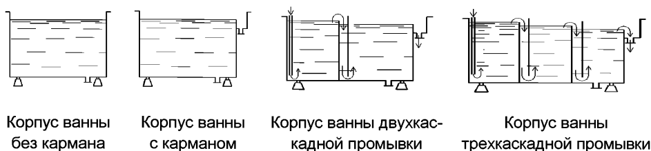
Рисунок 2.8 — Типы корпусов ванн
