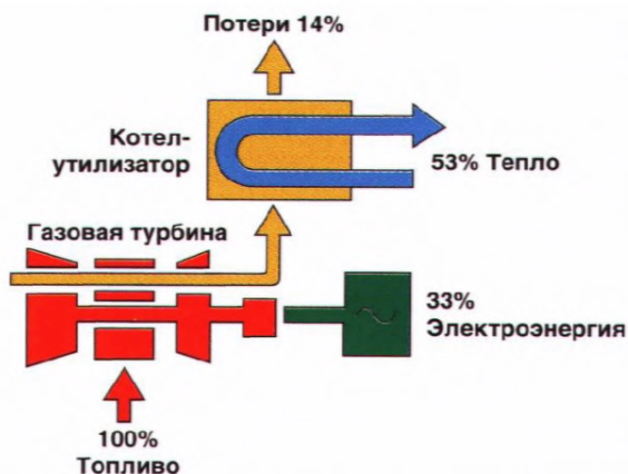
Рисунок 3.2 — Схема ГТУ-ТЭЦ
