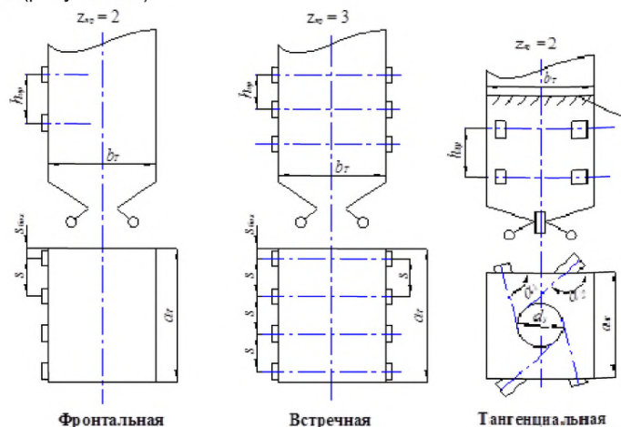
Рисунок 2.4 — Компоновка горелок
