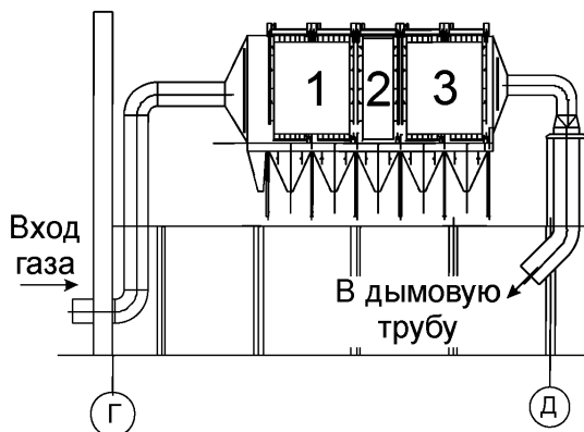
Рисунок 2.20 — Принципиальная схема комбинированного золоуловителя
