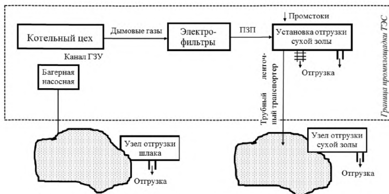
Рисунок 2.16 — Блок-схема системы отгрузки, транспортирования и складирования неотребоваанной части сухой золы на сухом золохранилище и шлака на гидрошлакоотвале Рефтинской ГРЭС.
