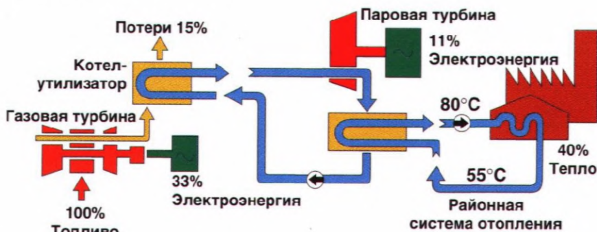
Рисунок 3.4 – Принципиальная схема ПГУ-ТЭЦ
