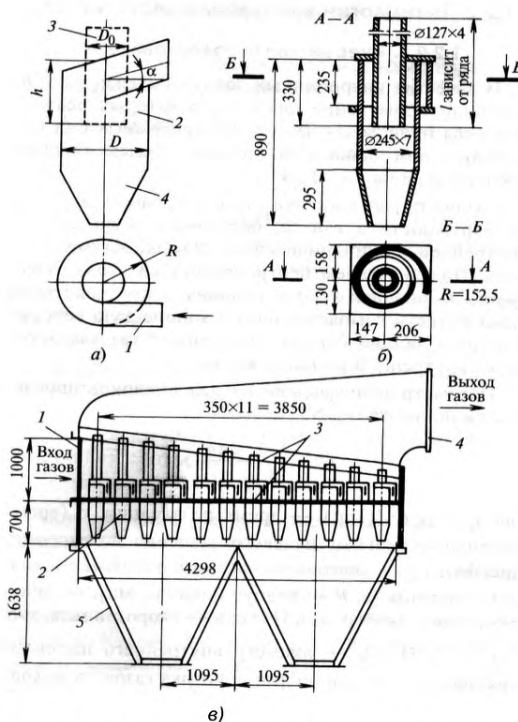
Рисунок 2.10 — Циклонные золоуловители
