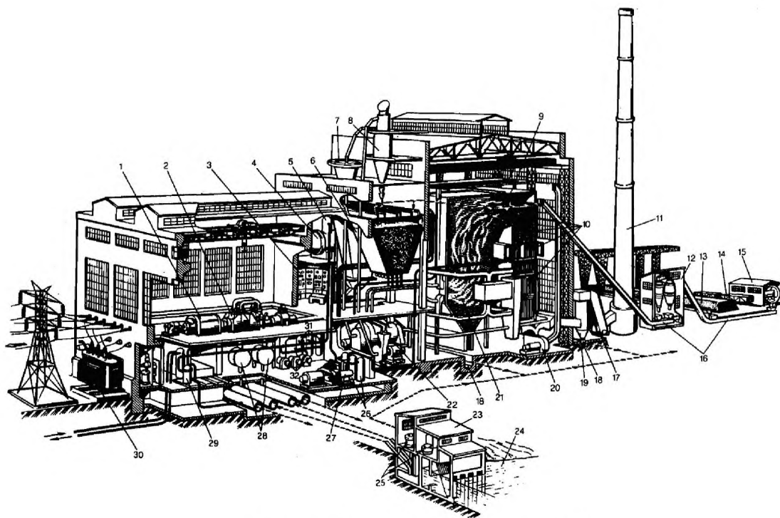
Рисунок 2.1 — Паротурбинная ТЭС
