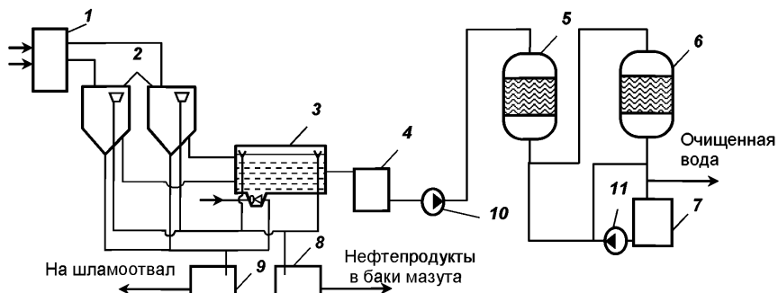
Рисунок 7.2 — Схема установки очистки сточных вод, загрязненных нефтепродуктами
