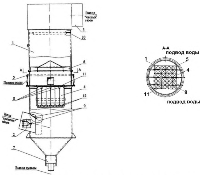
Рисунок 2.11 — Батарейный эмульгатор:
