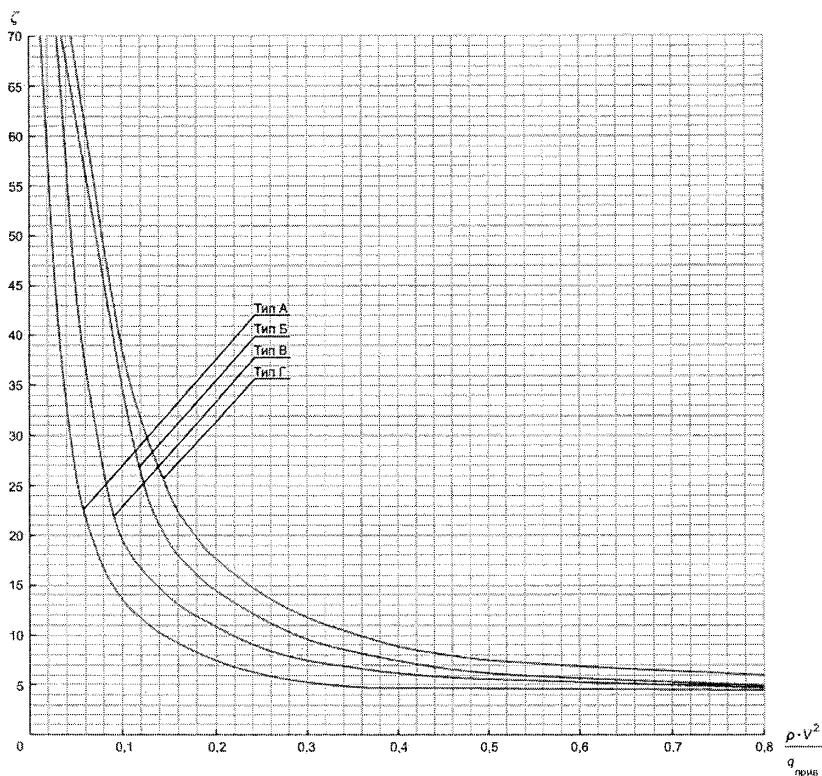
Рисунок 7 – Зависимость \zeta = f(\rho \cdot V^2 / q_{\text{прив}}) для затворов
