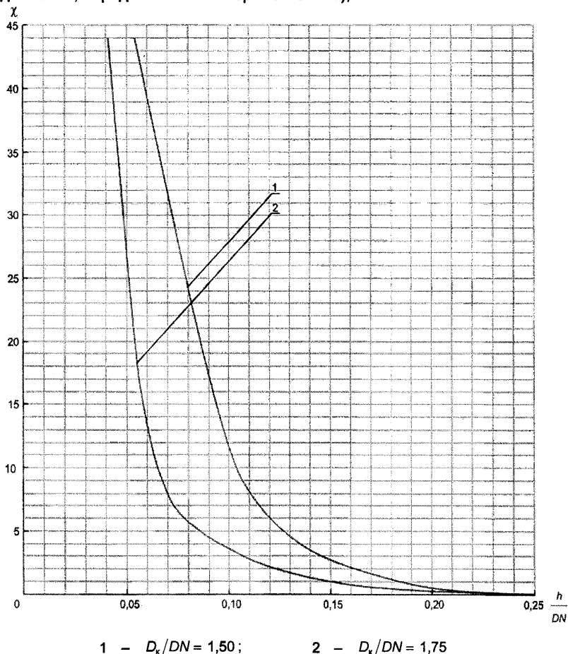
Рисунок 15 – Зависимость коэффициента подъемной силы от относительного хода \chi = f(h/DN) обратных клапанов
