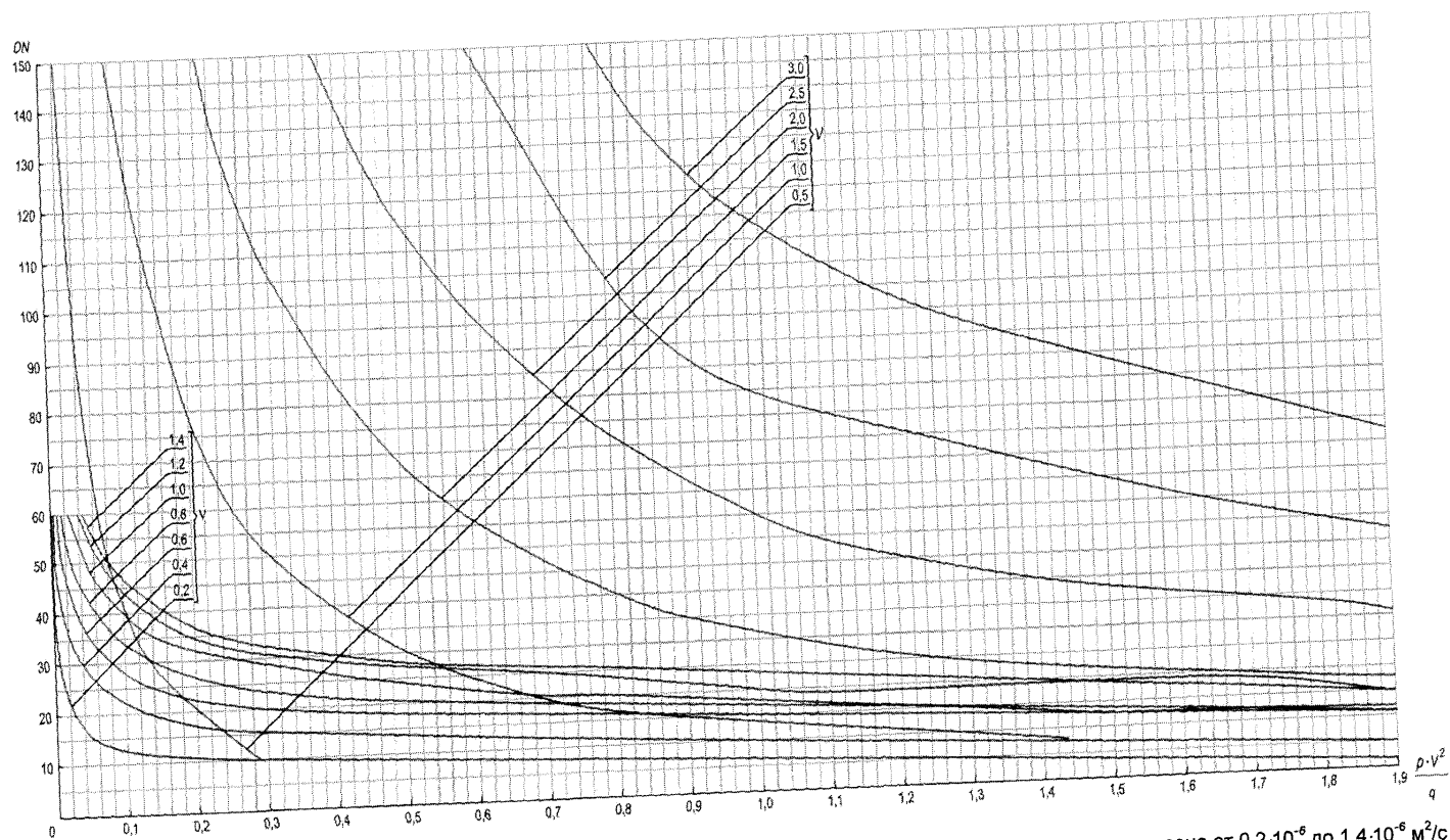
Рисунок 9 – Зависимость DN = f(\rho \cdot V^2 / q)_{0,1} для клапанов при \rho / \rho_s = 0,1 , V – в диапазоне от 0,5 до 3,0 м/с; \nu – в диапазоне от 0,2 \cdot 10^{-6} до 1,4 \cdot 10^{-6} м 2 /с
