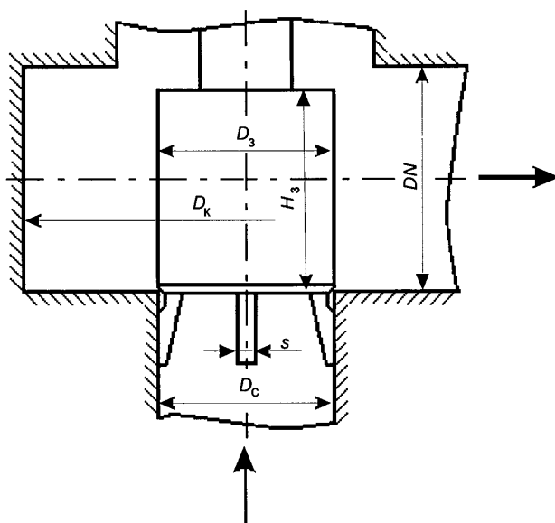
Рисунок 1 – Обратный подъемный угловой клапан, 3Эл с направлением в седле
