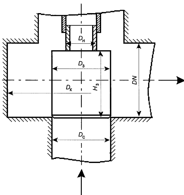
Рисунок 2 – Обратный подъемный угловой клапан, 3Эл с направлением в крышке
