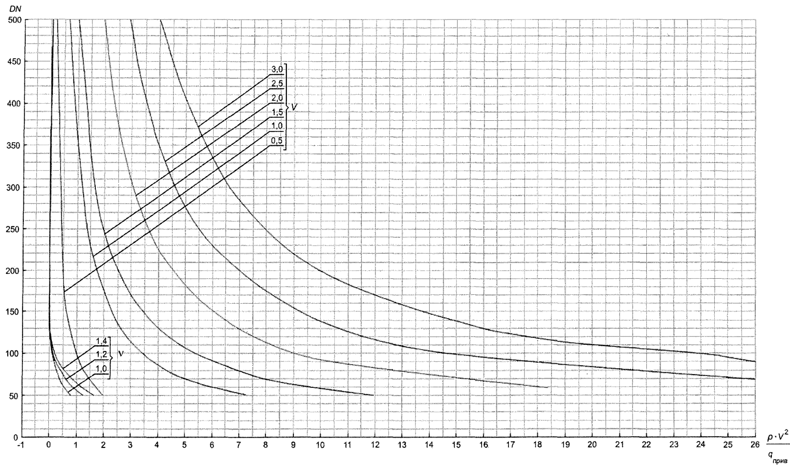
Рисунок 11 – Зависимость DN = f\left(\frac{\rho \cdot V^2}{q_{\text{прив}}}\right)_{0,1} для затворов с диском формы Б при \rho/\rho_3 = 0,1 ,
