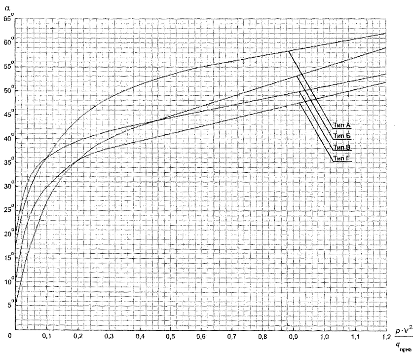
Рисунок 8 – Зависимость \zeta = f(\rho \cdot V^2 / q_{\text{прив}}) для затворов
