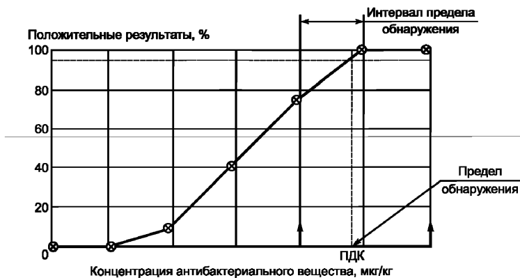
Рисунок 1 – Модель кривой содержание/сигнал для определения предела обнаружения
