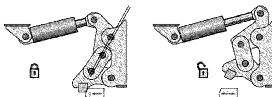
Рис. 17 Клиновое задрайка
