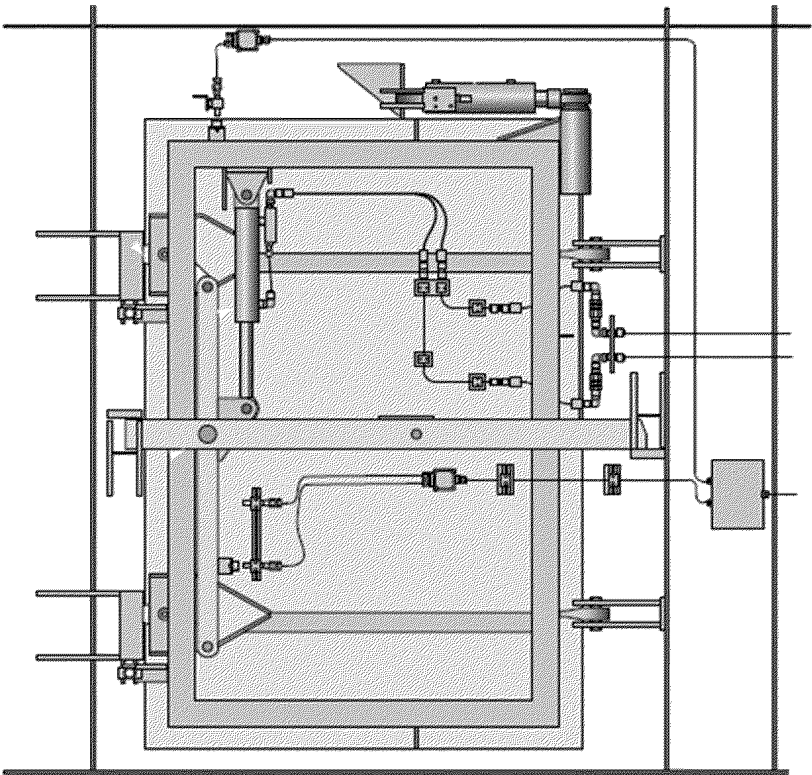
Рис. 36 Лопманская дверь – вид изнутри
