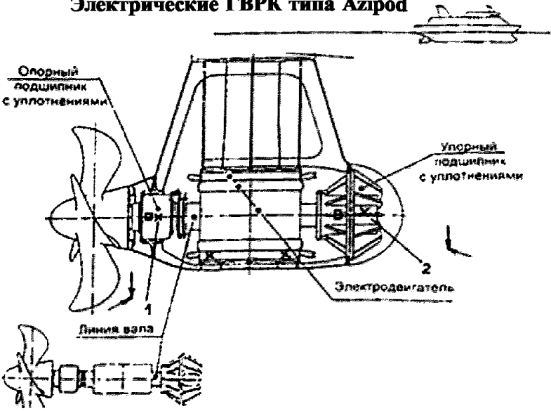
Электрические ГВРК типа Azipod
