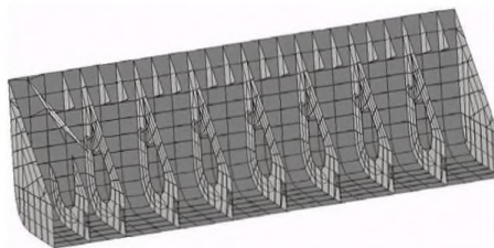
Рис. 2.2.3-2 Скуловые танки
