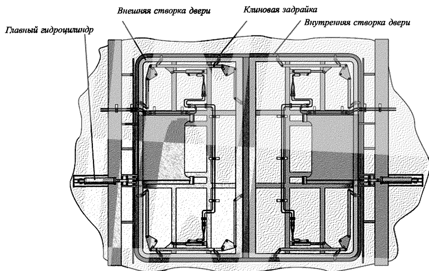
Рис. 32 Бортовая дверь – двухстворчатая, закрытое положение, вид изнутри
