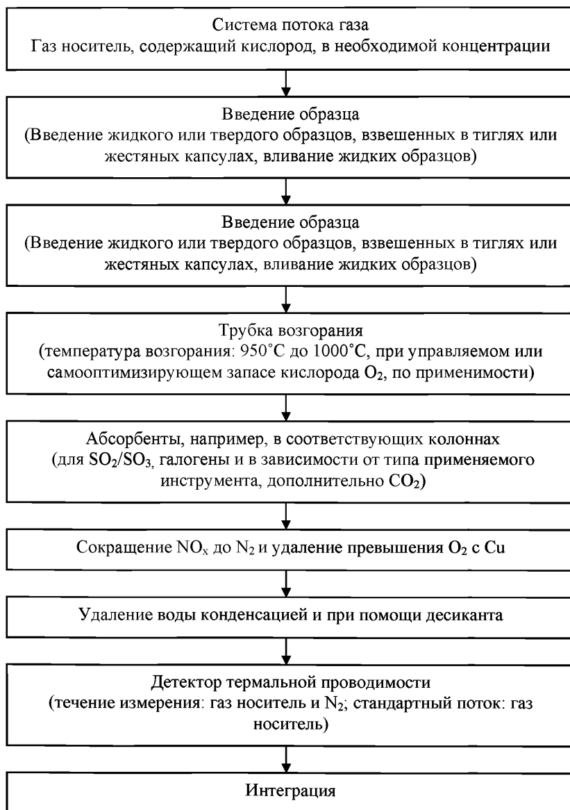
Рисунок А. 1 - Блок-схема базовой конструкции аппарата Дюмаса
