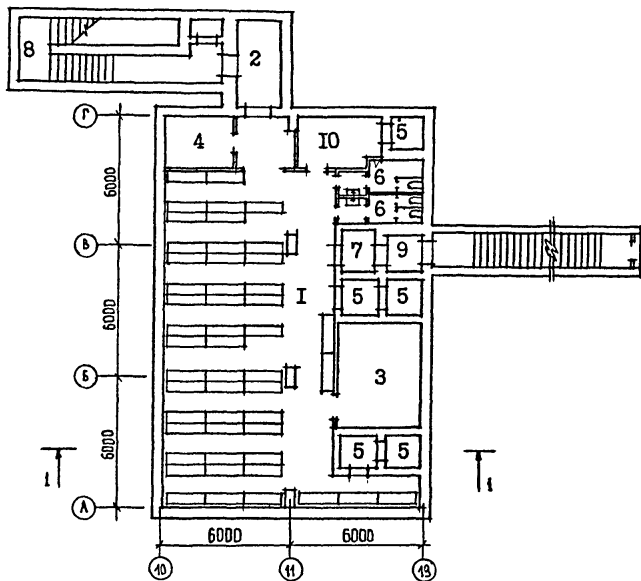
ЭКСПЛИКАЦИЯ ПОМЕЩЕНИЙ
