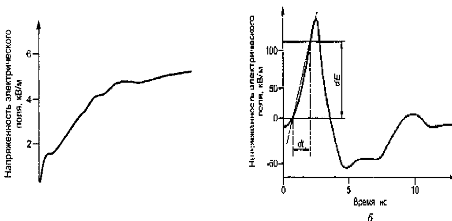
Рисунок В.1 — Типичные формы излучаемых импульсных полей
