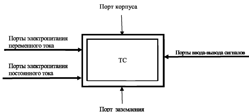
Рисунок 2 — Воздействие электромагнитных помех на порты ТС
