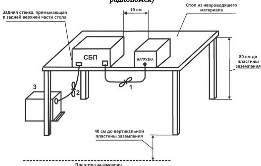
Рисунок 3 — Рабочее место для испытаний напольных СБП (измерение напряжения радиопомех)
