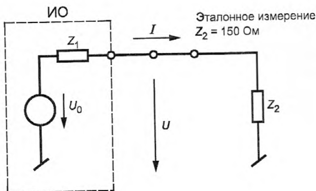
Рисунок F.1 – Основная схема рассмотрения норм РП при заданном значении суммарного общего несимметричного полного сопротивления, равном 150 Ом
