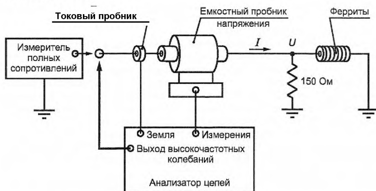
Рисунок F.4 – Установка для измерения полного сопротивления резистора сопротивлением 150 Ом и ферритов
