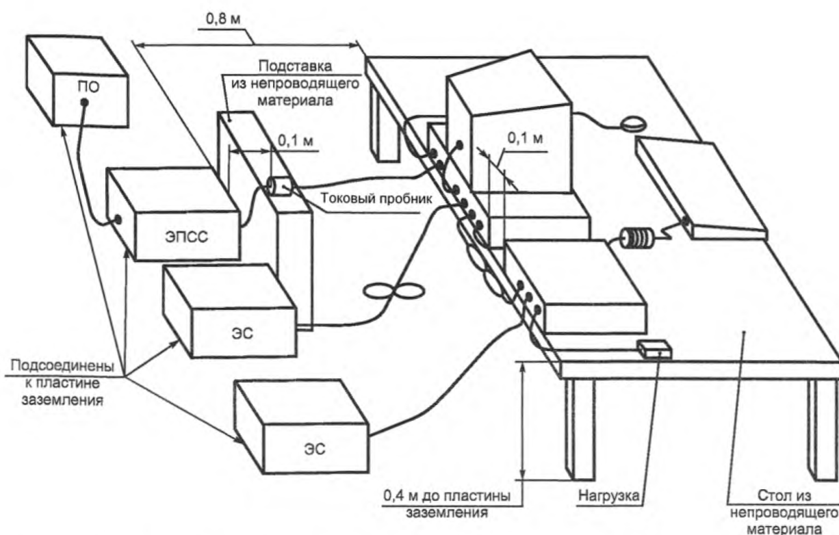
Рисунок 7 – Пример расположения настольного оборудования при испытаниях (измерение кондуктивных РП – вариант 1б)
