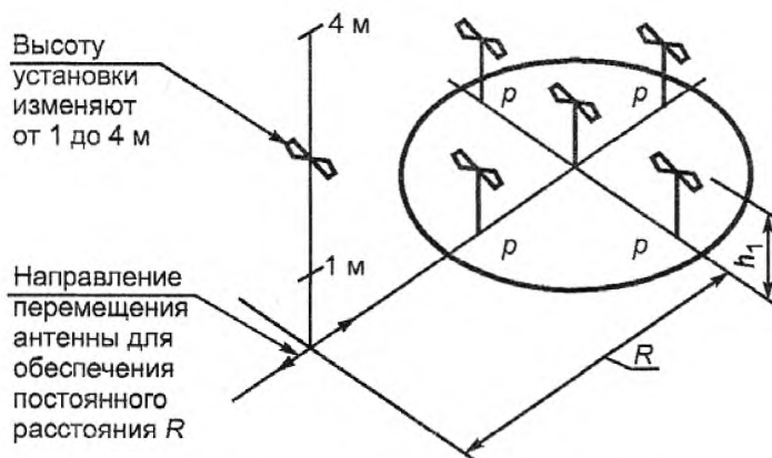
Рисунок А.1а – Расположение антенн при измерении затухания альтернативной площадки NSA (вертикальная поляризация)
