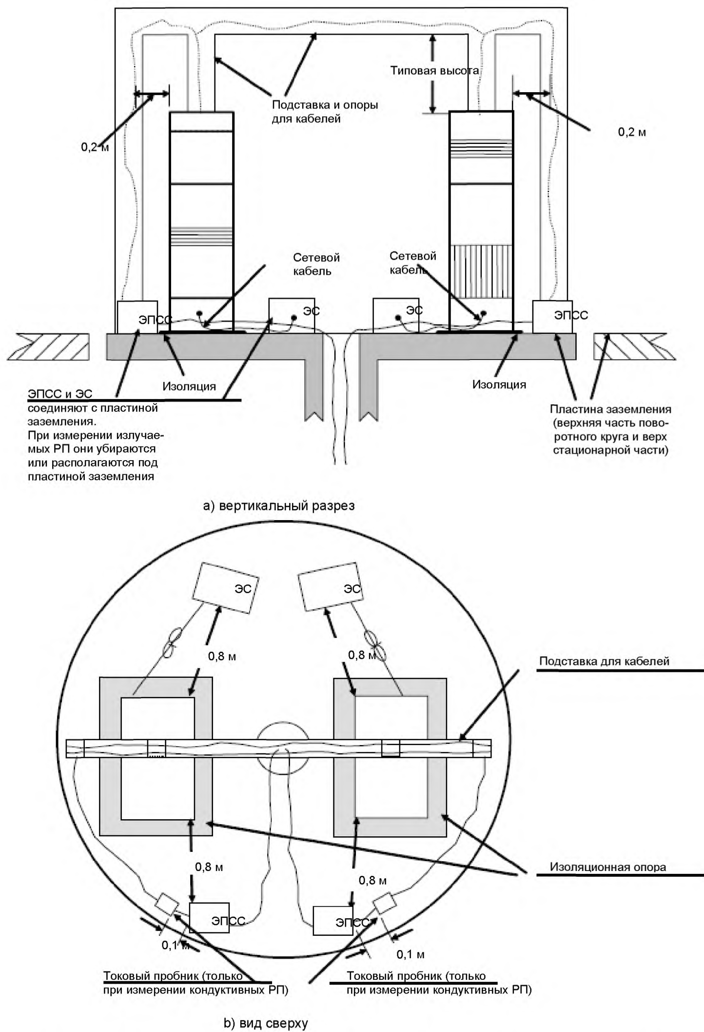
Рисунок 12 – Расположение напольного оборудования с вертикальным подъемником и воздушными кабелями (измерение излучаемых и кондуктивных РП)
