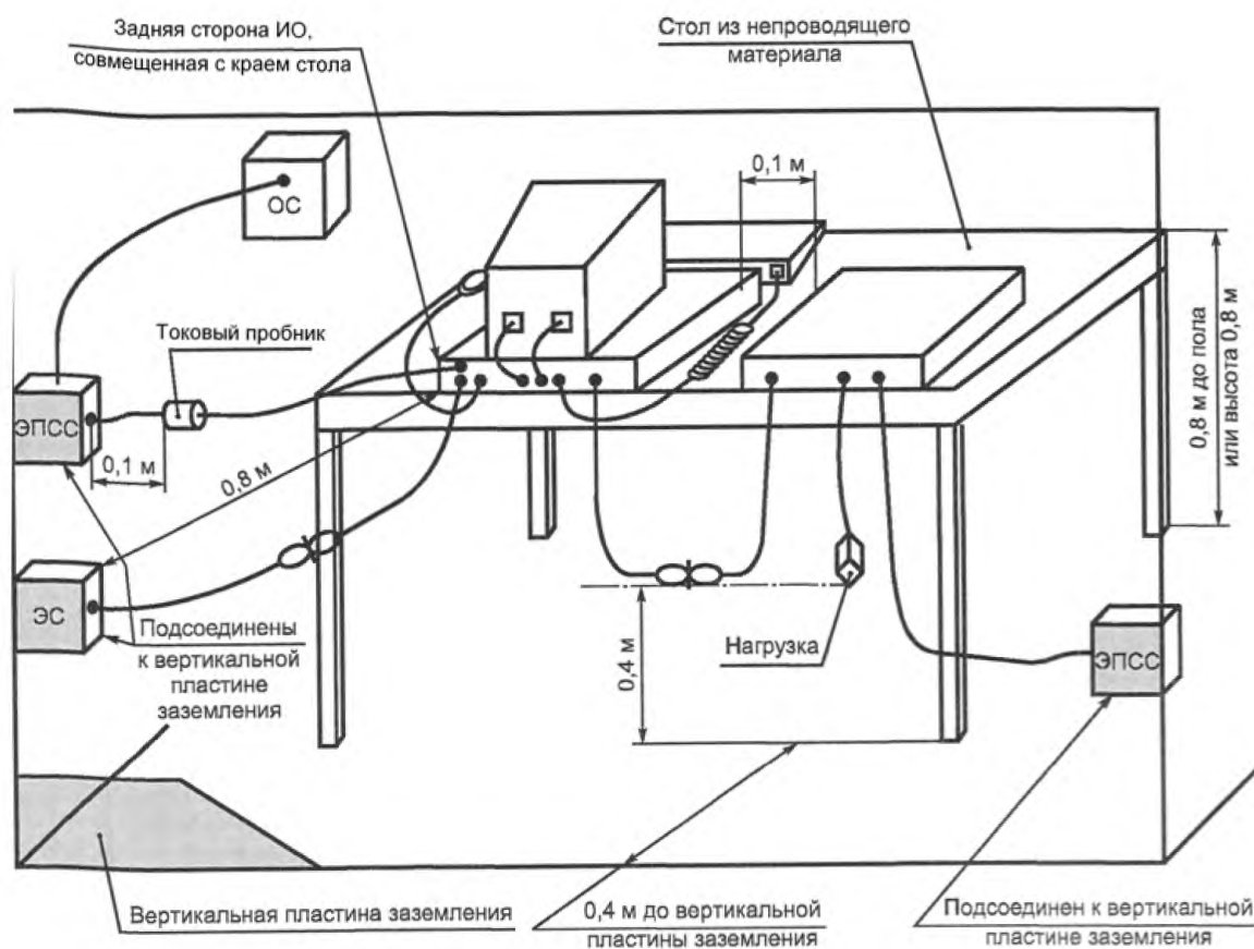
Рисунок 6 – Пример расположения настольного оборудования при испытаниях (измерение кондуктивных РП – вариант 1б)
