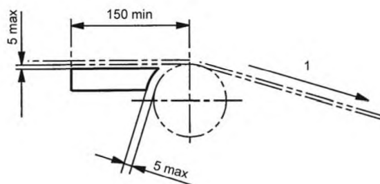
1 – направление движения ленты
