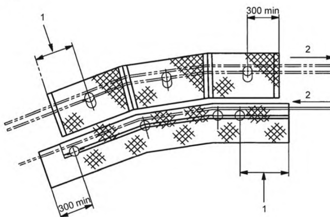
1 – расстояние a (см. таблицу 1); 2 – направление движения ленты
