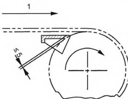
Рисунок 9 а) – Конструкция из стального профиля
