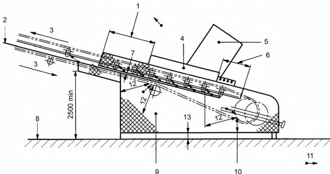
Рисунок 5 – Типовые ограждения переднего концевой барабана и расположение переходных роликоопор конвейера
