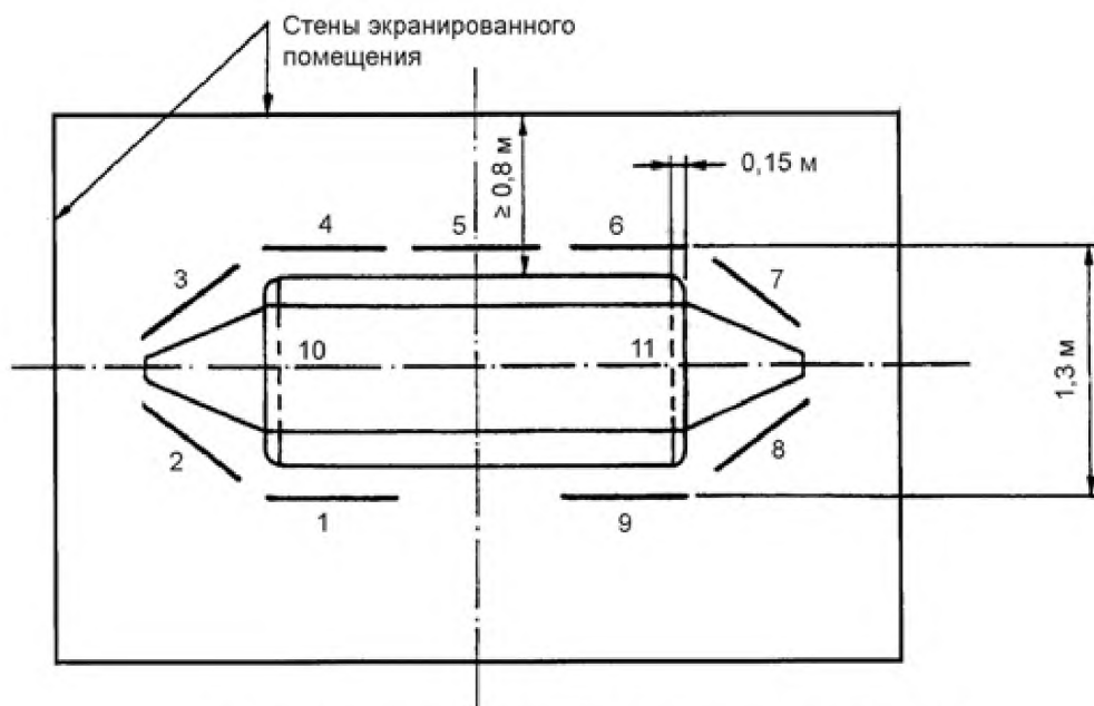
Рисунок 9 – Пример компоновки открытой полосковой ТЕМ-камеры в сочетании с радиопоглощающими пластинами внутри экранированного помещения размерами 3 \times 3,5 м
