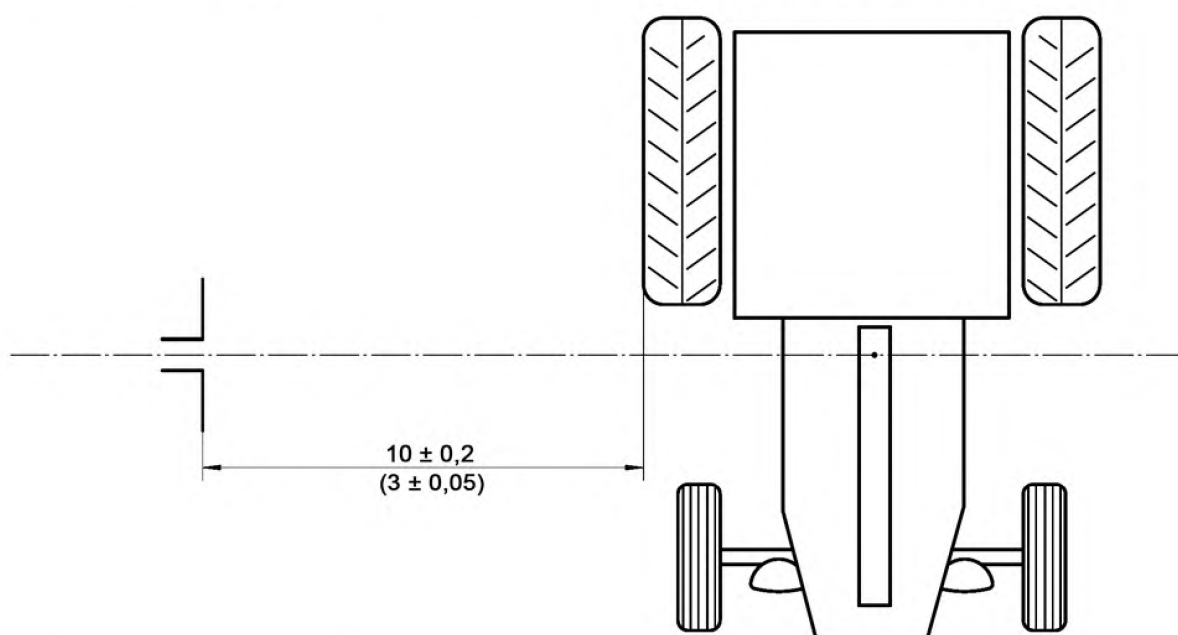
б) Расположение дипольной антенны для измерения излучения с горизонтальной поляризацией
