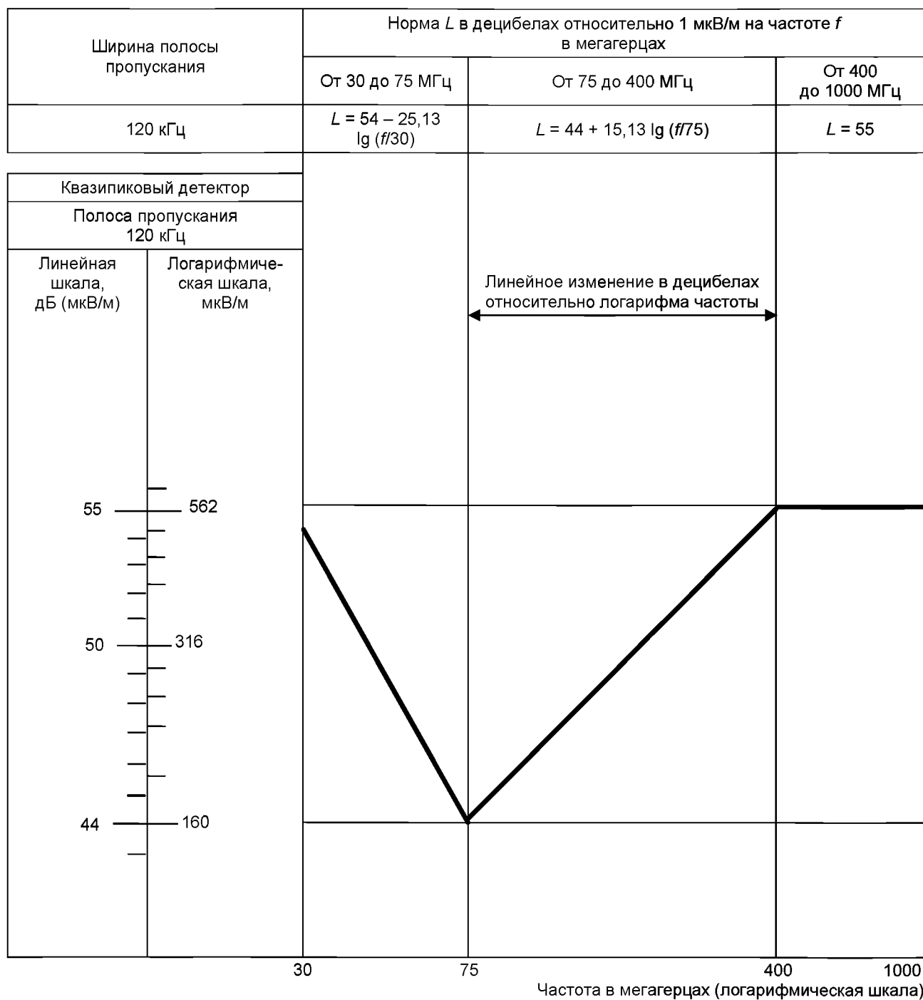
Рисунок А.6 – Нормы узкополосного излучения для сборочных узлов
