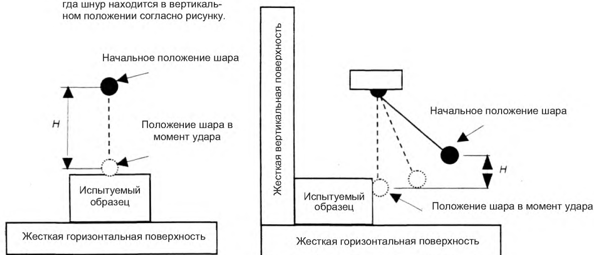
Рисунок 12 – Метод испытаний на ударостойкость
