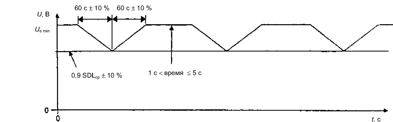
Рисунок 10 – Испытание на медленное изменение напряжения питания
