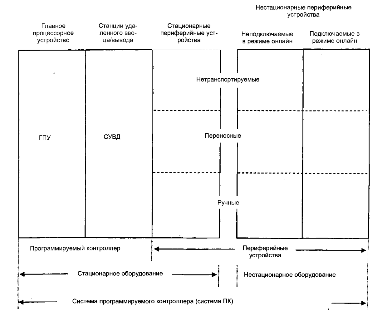
Рисунок А.1 – Система программируемого контроллера (система ПК)
