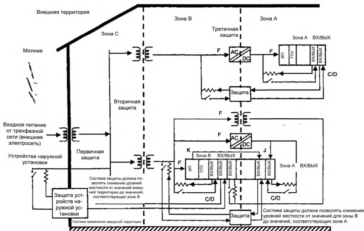
Рисунок 11 – Зоны устойчивости к электромагнитным помехам
