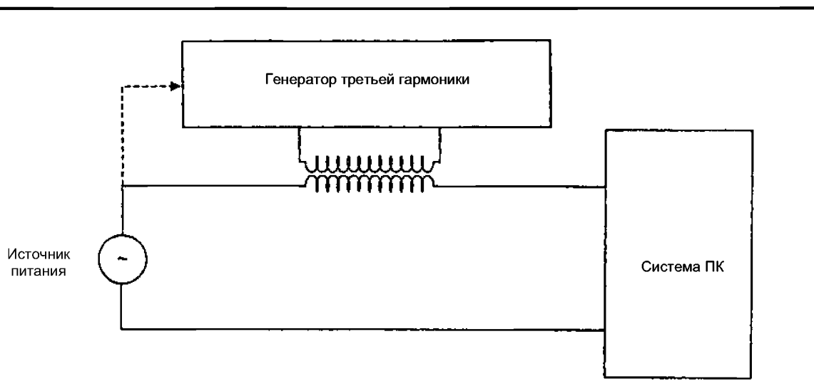
Рисунок 7 – Испытание на устойчивость к напряжению третьей гармоники
