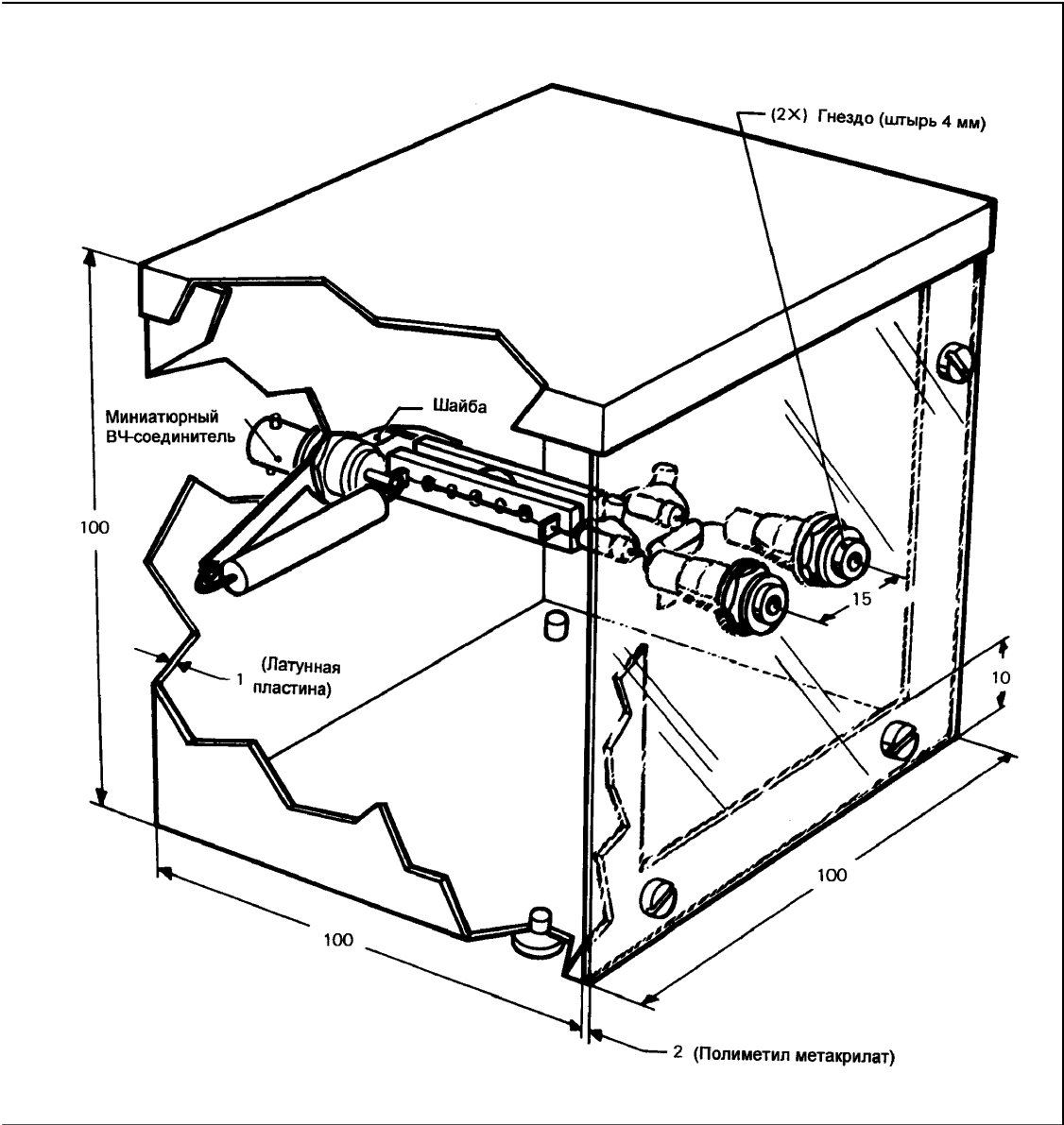
Рисунок А.2d – Конструкция трансформатора
