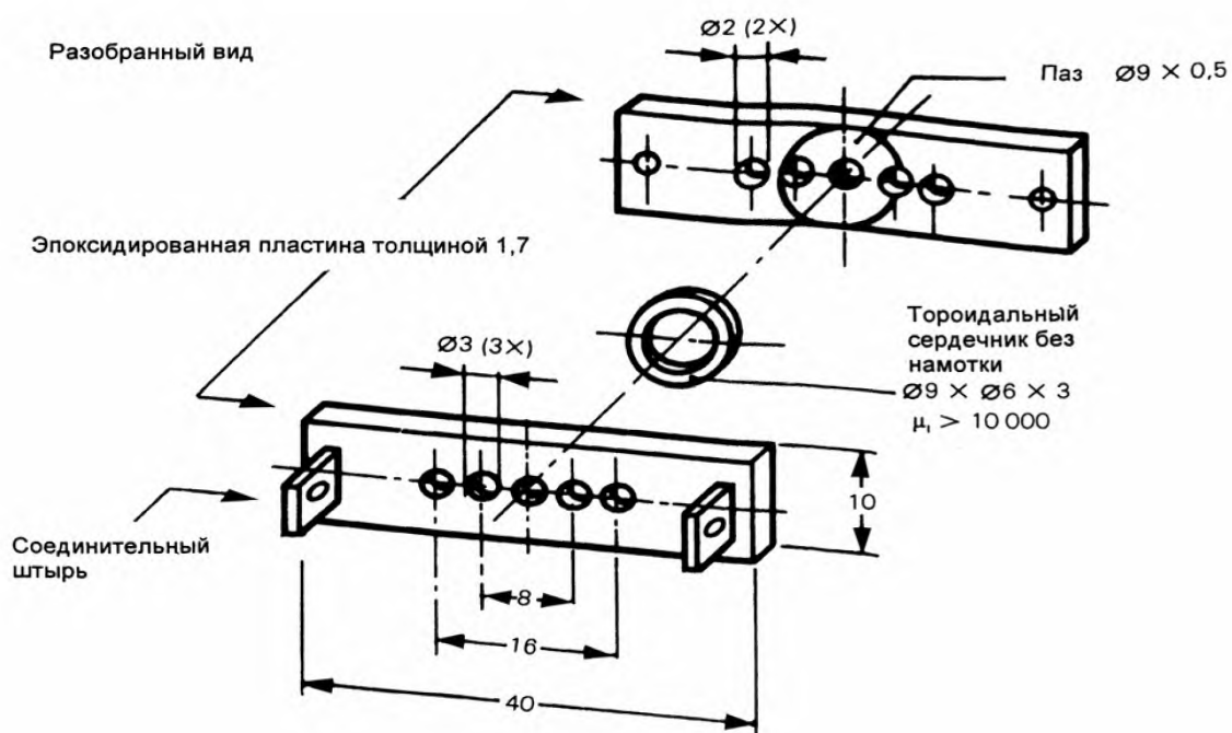
Рисунок А.2b – Детали конструкции сердечника трансформатора
