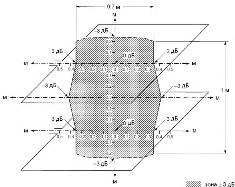
Рисунок В.4 – Зона \pm 3 дБ магнитного поля, создаваемого двумя индукционными катушками квадратной формы (с длиной стороны 1 м), разнесенными на расстояние 0,6 м, в центральной ортогональной плоскости (компонента, перпендикулярная плоскости катушки)
