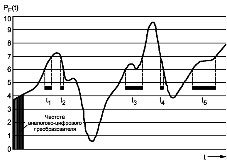
Рисунок 2а — Уровень фликера как функция времени
