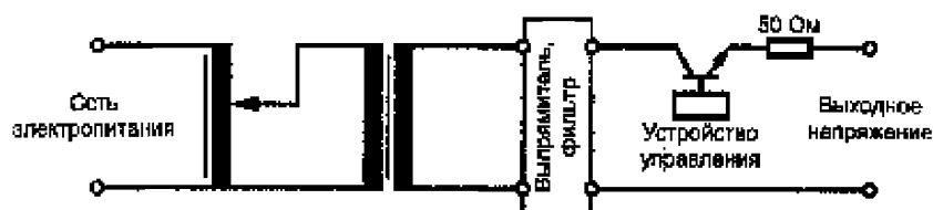
Рисунок 3- Схема ИГ постоянного тока
