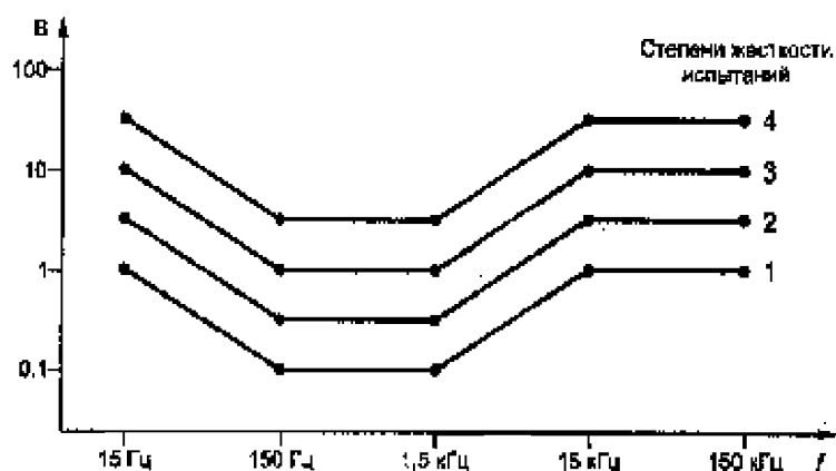
Рисунок 2- Зависимость испытательного напряжения от частоты
