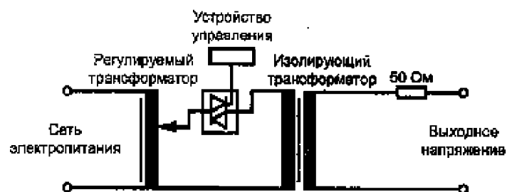
Рисунок 4- Схема ИГ на частоте 50 Гц
