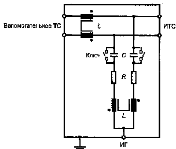
Рисунок 4- Схема ИГ на частоте 50 Гц
