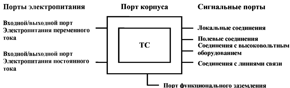
Рисунок 1 - Порты ТС
