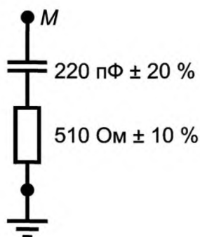
а) Элемент RC
