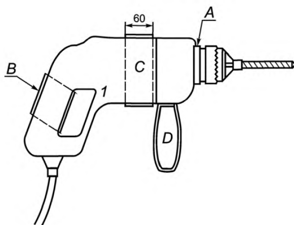
а) Элемент RC
