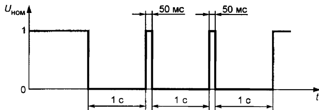
Рисунок В.1 - Прерывания напряжения AU = 100\% , продолжительность 1 с
