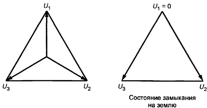
Рисунок С.2 – Напряжения на испытуемом источнике
