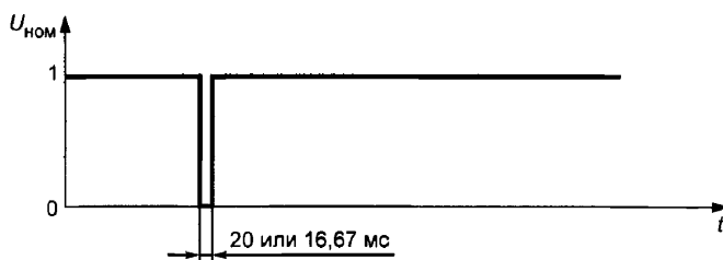
Рисунок В.2 - Прерывания напряжения AU = 100\% , в течение одного цикла при номинальной частоте
