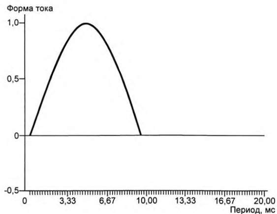
Рисунок А.2 — Форма тока при однополупериодном выпрямлении
