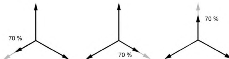
Рисунок 4a) – Испытание «фаза – фаза» в трехфазной системе электропитания
