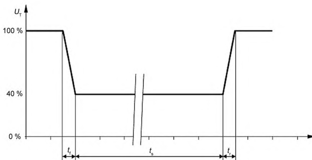
Рисунок 1а) – Провал напряжения. График синусоидального колебания провала напряжения до 70 % U_T
