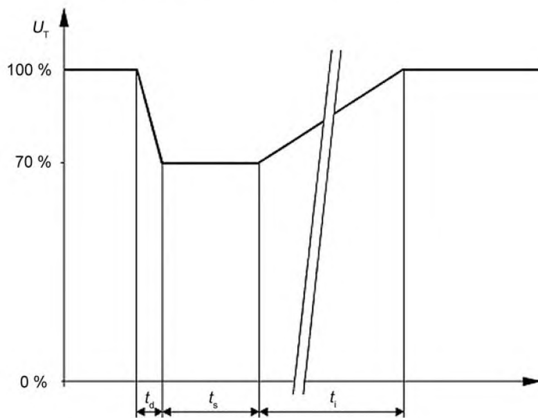
Рисунок 2 – Кратковременное прерывание
