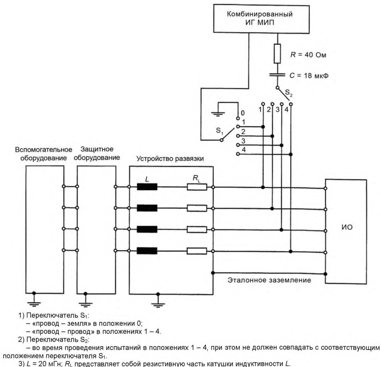
Рисунок 11 – Пример организованного места для испытаний при подаче МИП по схеме «провод – провод» и «провод – земля» с использованием емкостной связи на незранированные соединительные линии (в соответствии с 7.3)
