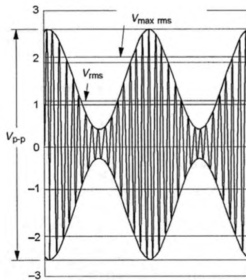
б) модулированный радиочастотный сигнал при глубине модуляции 80 %: пиковое значение напряжения V_{p-p} = 5,1 \text{ В} ; среднеквадратическое значение напряжения – V_{rms} = 1,15 \text{ В} ; максимальное среднеквадратическое – значение напряжения V_{max rms} = 1,8 \text{ В}
