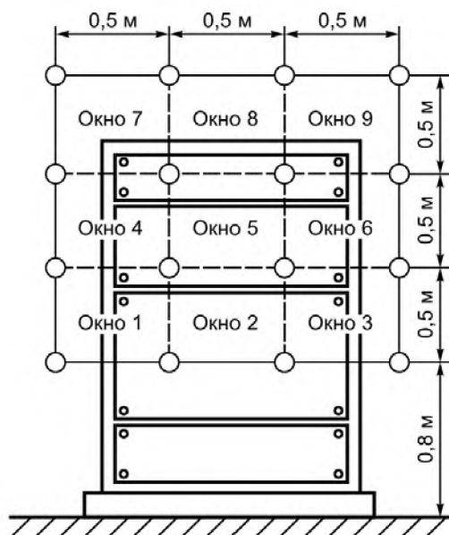
Рисунок Н.1б – Пример деления калиброванной плоскости однородного поля на окна размером 0,5 \times 0,5 м для напольного оборудования
