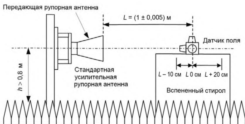
Рисунок І.3 – Испытательная установка для проведения проверки камеры
