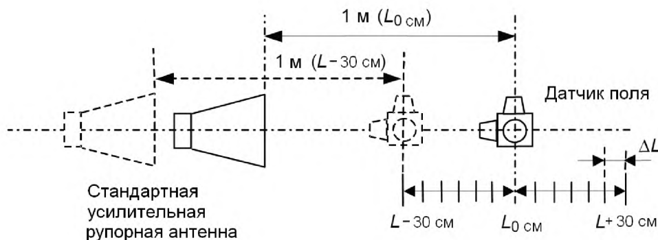
Рисунок І.7 – Расположение передающей антенны и датчика поля при проведении проверки камеры
