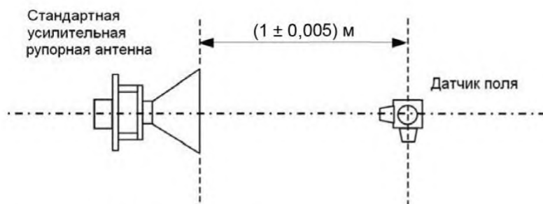
Рисунок І.10 – Расположение датчика поля при калибровке (вид сверху)
