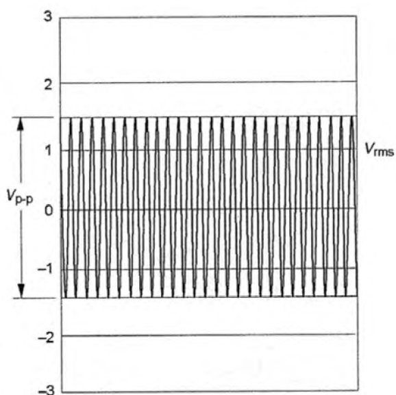
а) немодулированный радиочастотный сигнал: пиковое значение напряжения V_{p-p} = 2,8 \text{ В} ; среднеквадратическое значение напряжения – V_{rms} = 1,0 \text{ В}
