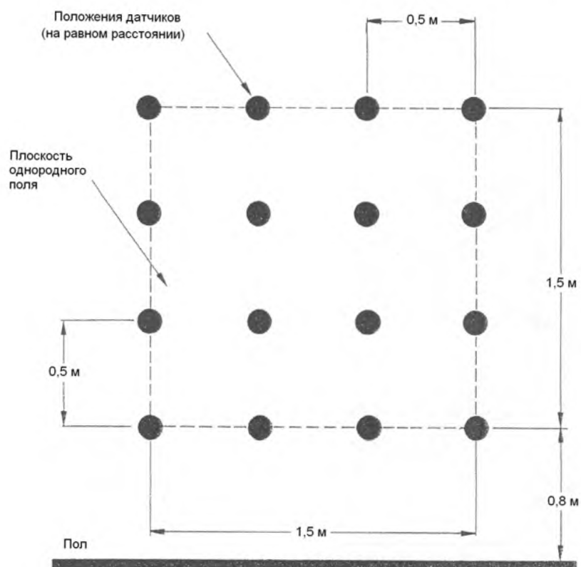
Рисунок 4 – Размеры плоскости однородного поля
