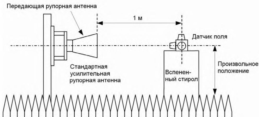
Рисунок І.6 – Пример расположения антенны и датчика
