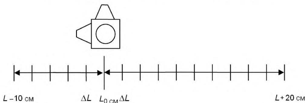
Рисунок І.4 – Позиция датчика при определении КСВН камеры при изменении с шагом \Delta L
