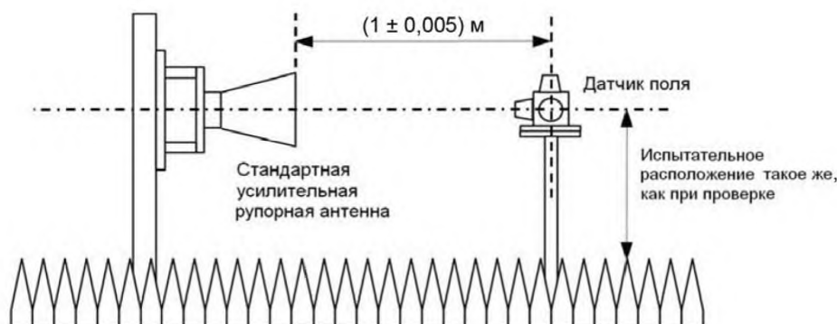
Рисунок І.9 – Расположение датчика поля при калибровке
