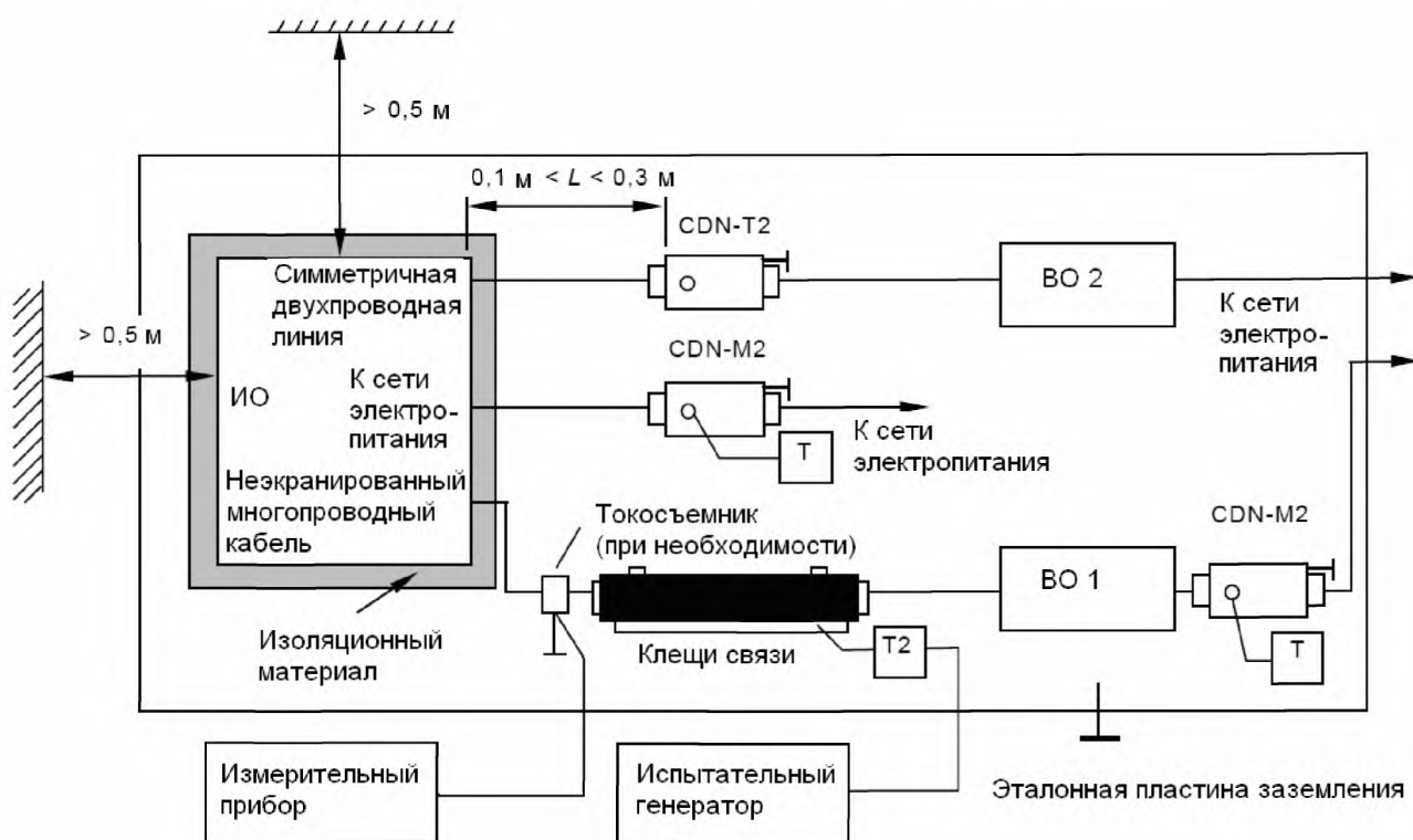
Рисунок А.6 – Общая схема расположения оборудования для испытаний с использованием клещей связи
