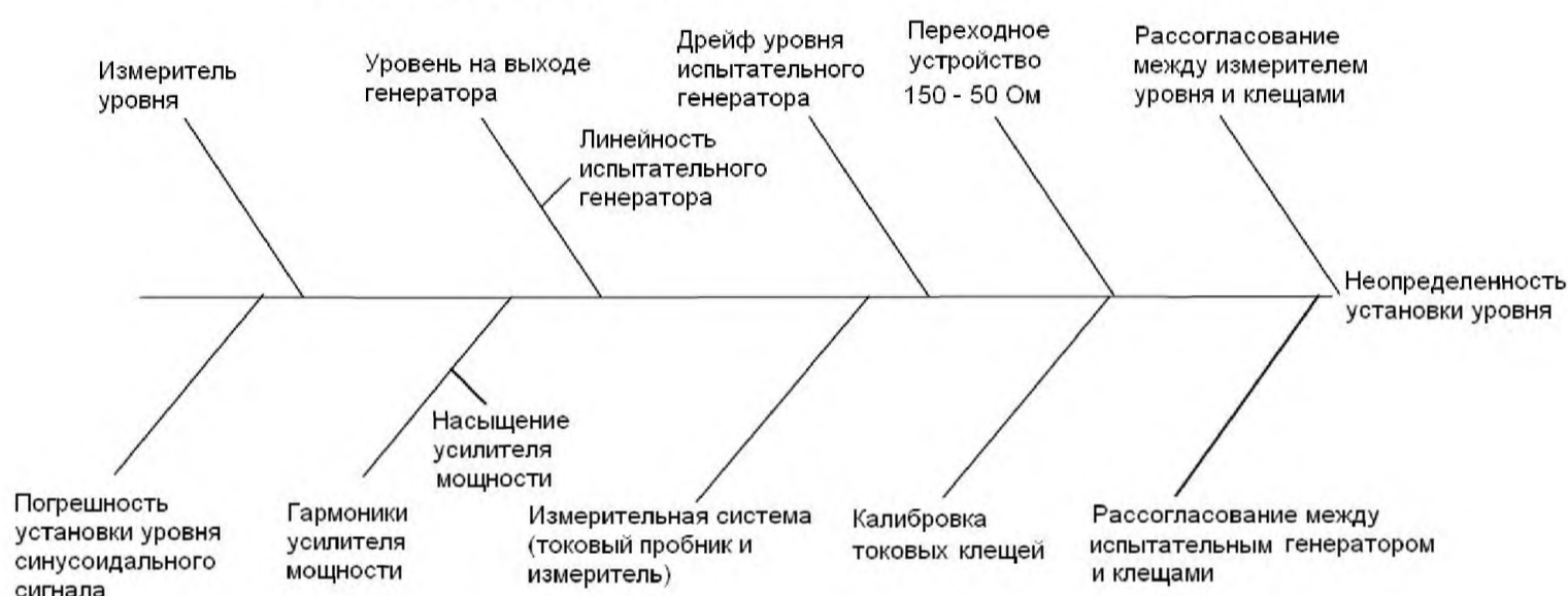
Рисунок G.3 – Пример влияний на установку уровня для метода испытаний с использованием токовых клещей
