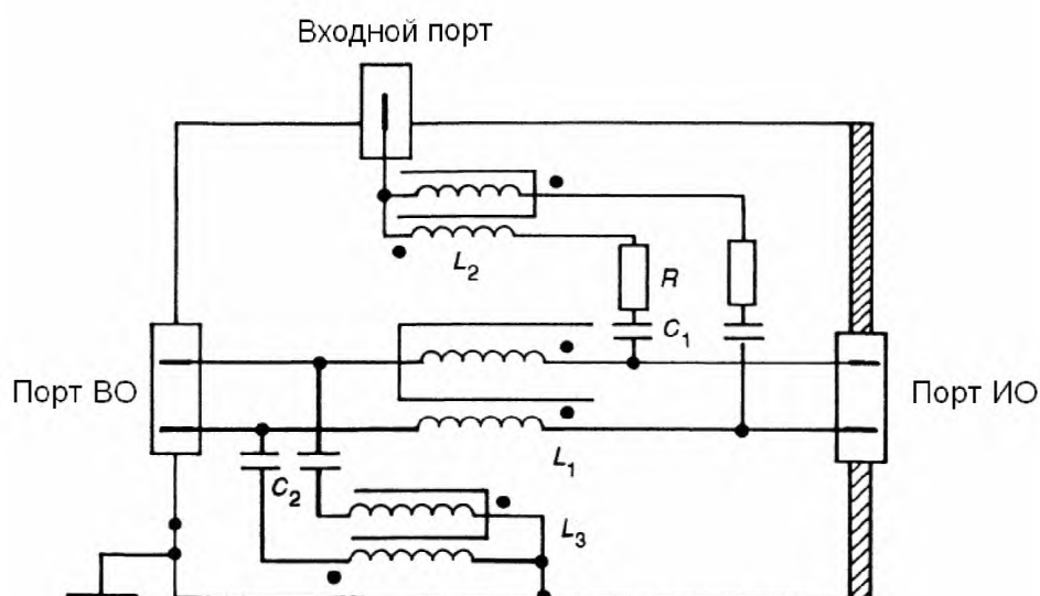
Рисунок D.3 – Пример упрощенной схемы УСР типа CDN-AF2, применяемого при вводе помехи в неэкранированные несимметричные линии (см. 6.2.1.3)
