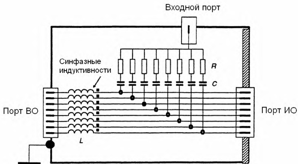
Рисунок D.5 – Пример упрощенной схемы УСР типа CDN-T4, применяемого при вводе помехи в незранированные симметричные пары (четырепроводную линию) (см. 6.2.1.2)
