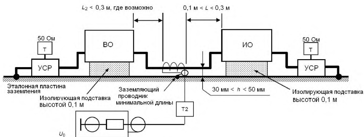
Рисунок 5 – Принцип связи и развязки
