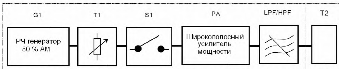
Рисунок 2 – Испытания на устойчивость к радиочастотным кондуктивным помехам
