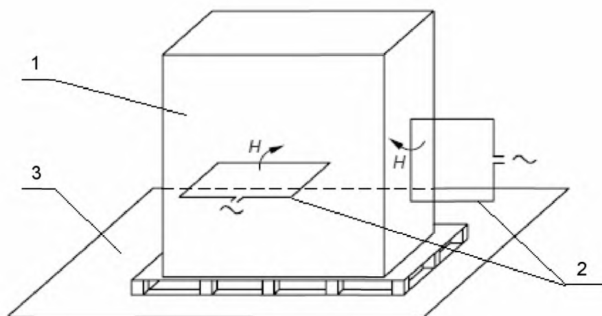
Рисунок 6 – Схема проверки восприимчивости ИО на устойчивость к магнитному полю промышленной частоты методом приближения с использованием индукционной катушки с размером витка 1 × 1 м
