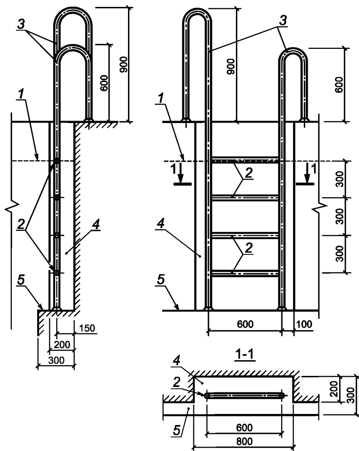
1 — уровень воды; 2 — ступени; 3 — разновысокие поручни; 4 — ниша; 5 — уступ для отдыха
