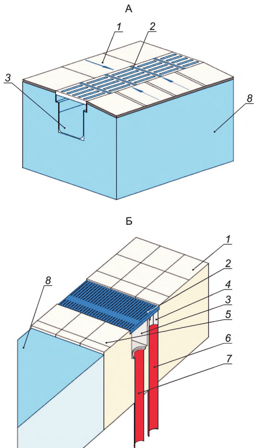
А — Схема переливного желоба с объединенным лотком; Б — Схема переливного желоба с раздельным сбором воды; 1 — обходная дорожка; 2 — декоративная решетка; 3 — лоток для сбора воды; 4 — лоток для сбора воды с отводом в канализацию; 5 — пространство между желобом и отвесом ванны; 6 — отвод воды в канализацию из отдельного лотка; 7 — отвод воды в систему рециркуляции; 8 — уровень воды
