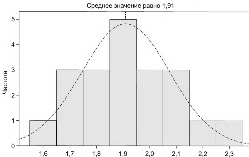
Рисунок 2 — Распределение результатов повторных измерений
