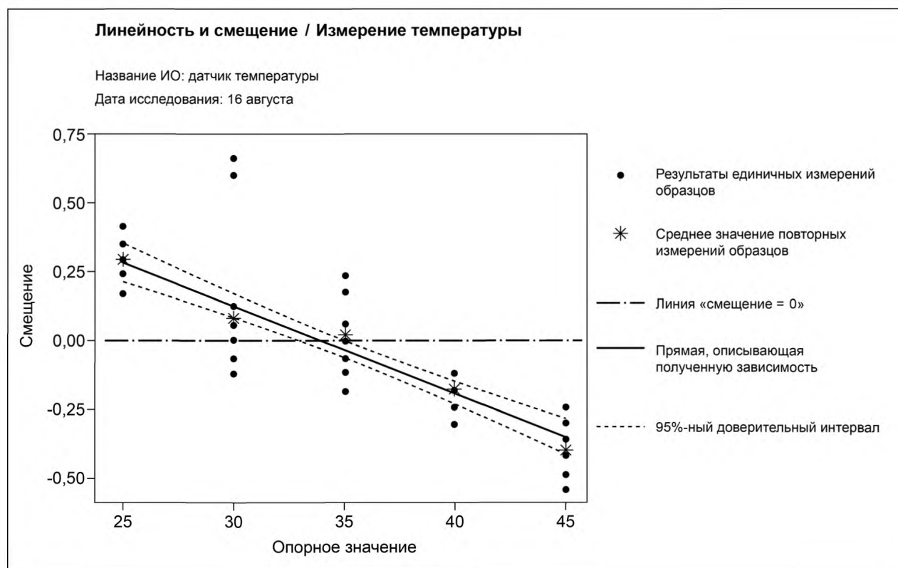
Рисунок Е.1 — Линейность ПИ
