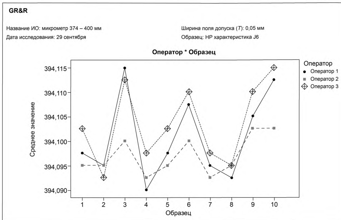
Рисунок Г.2 — Сравнение операторов
