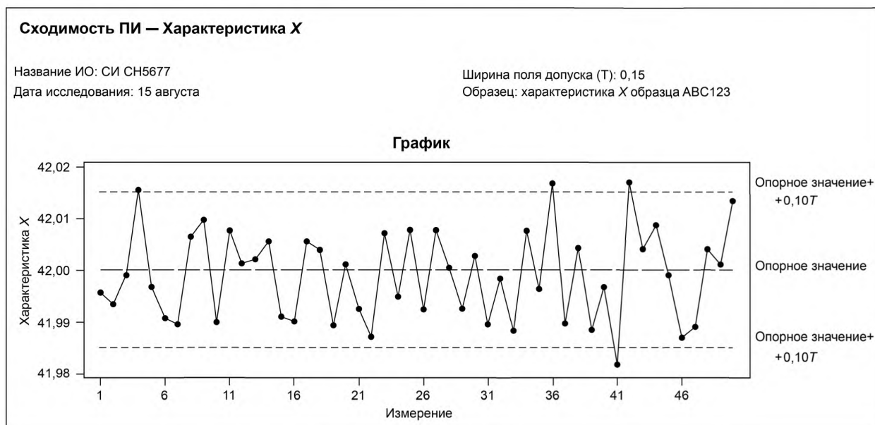
Рисунок В.1 — Анализ сходимости ПИ
